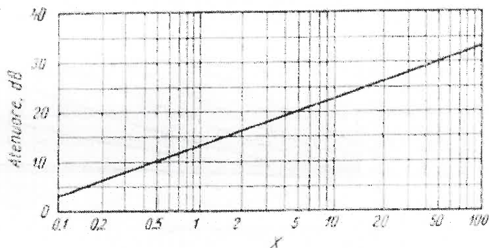
Fig. 4.1. Atenuarea zgomotului datorit ecranelor protectoare în aer liber.
