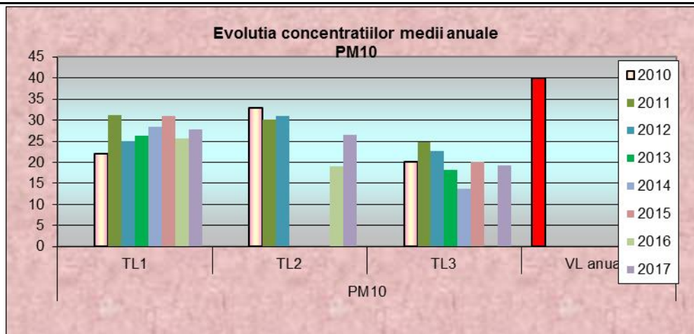
Fig.15 - Concentrații medii anuale PM10
