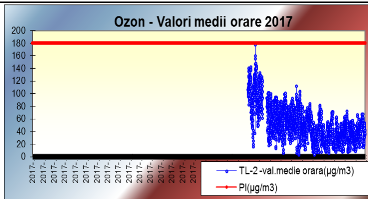
Fig. 6. Concentrații medii orare O3-2017
