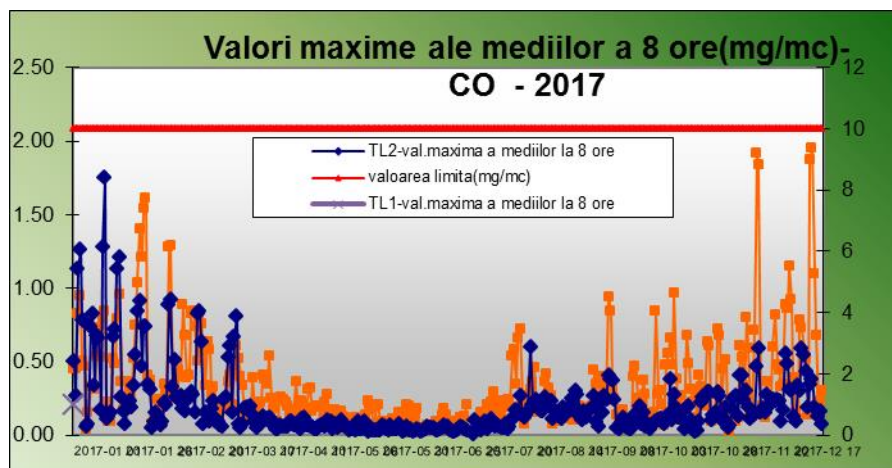
Fig. 9 Valori maxime zilnice a mediilor la 8 ore – CO – 2017
