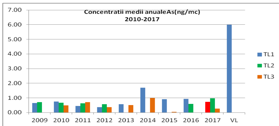
Fig.20 - Concentrații medii anuale As
