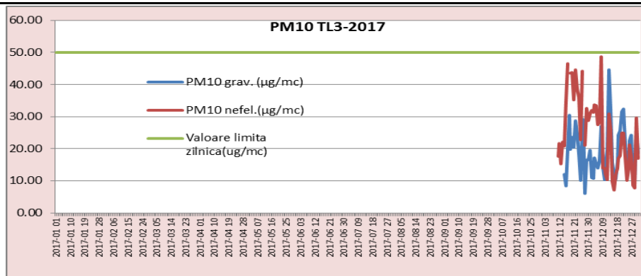
Fig.14 TL3:Concentrații medii zilnice PM10 grav.-2017
