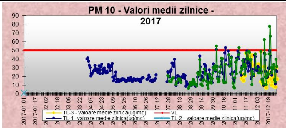
Fig.11 Concentrații medii zilnice PM10 nefelometric -2017
