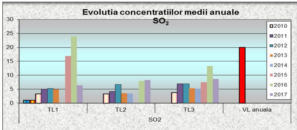
Fig. 5 Valorile concentrației medii anuale de SO 2
