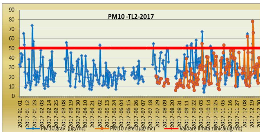
Fig.13 TL2: Concentrații medii zilnice PM10 grav.-2017
