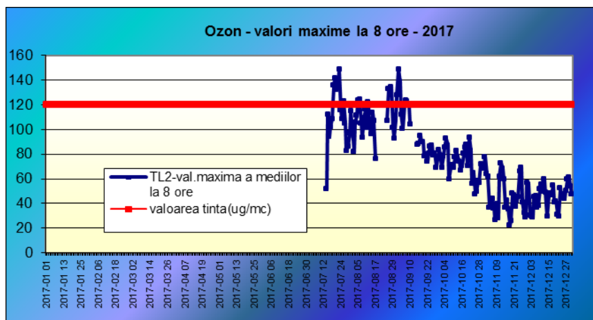
Fig. 7 Valori maxime zilnice a mediilor la 8 ore – O3 – 2017
