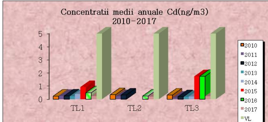
Fig.21 - Concentrații medii anuale Cd
