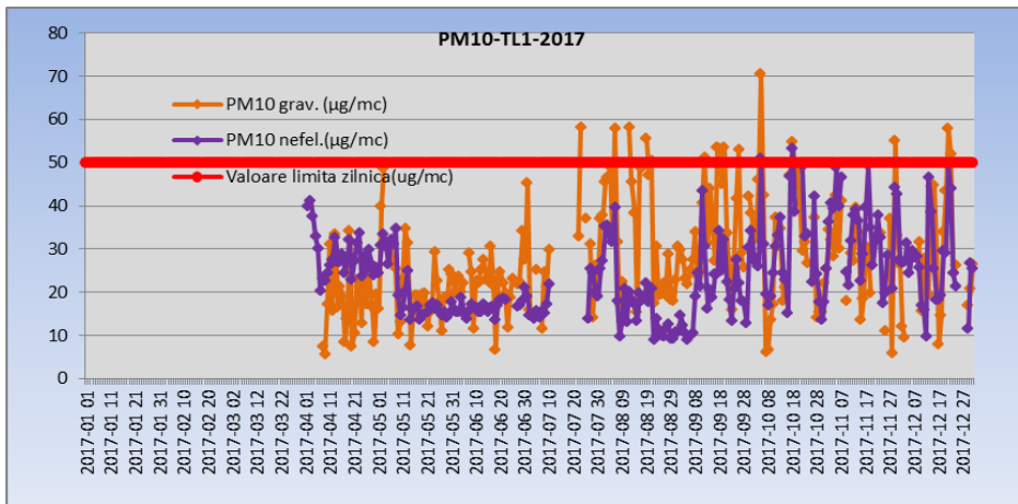
Fig.12 TL1: Concentrații medii zilnice PM10 grav. - 2017
