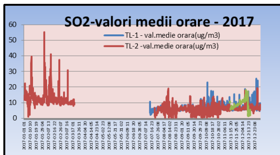
Fig. 3 Concentrații medii orare SO2 -2017
