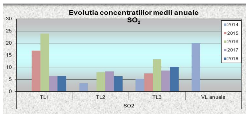
Fig. 5 Valorile concentrației medii anuale de SO 2
