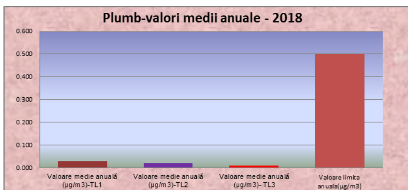
Figura nr.16 Valori medii anuale – plumb – 2018
