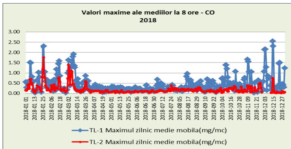
Fig. 9 Valori maxime zilnice a mediilor la 8 ore – CO – 2018
