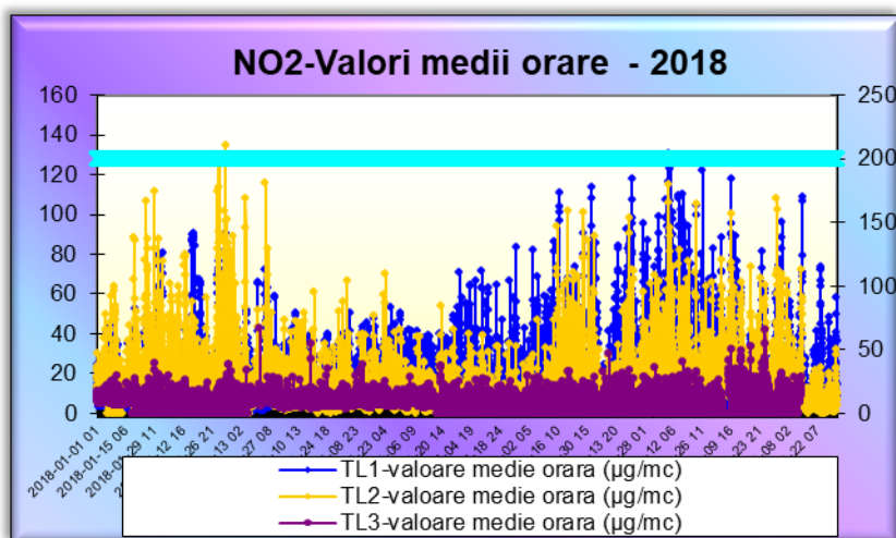
Fig. 1 Concentrații medii orare NO2 -2018
