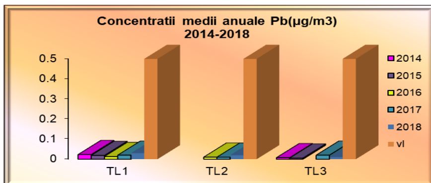
Fig.19 - Concentrații medii anuale Pb
