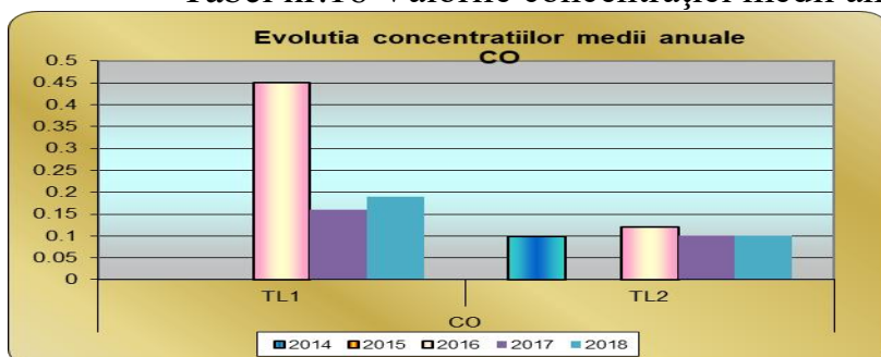
Fig. 10 Valorile concentrației medii anuale de CO
