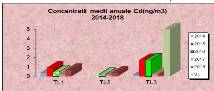
Fig.21 - Concentrații medii anuale Cd
