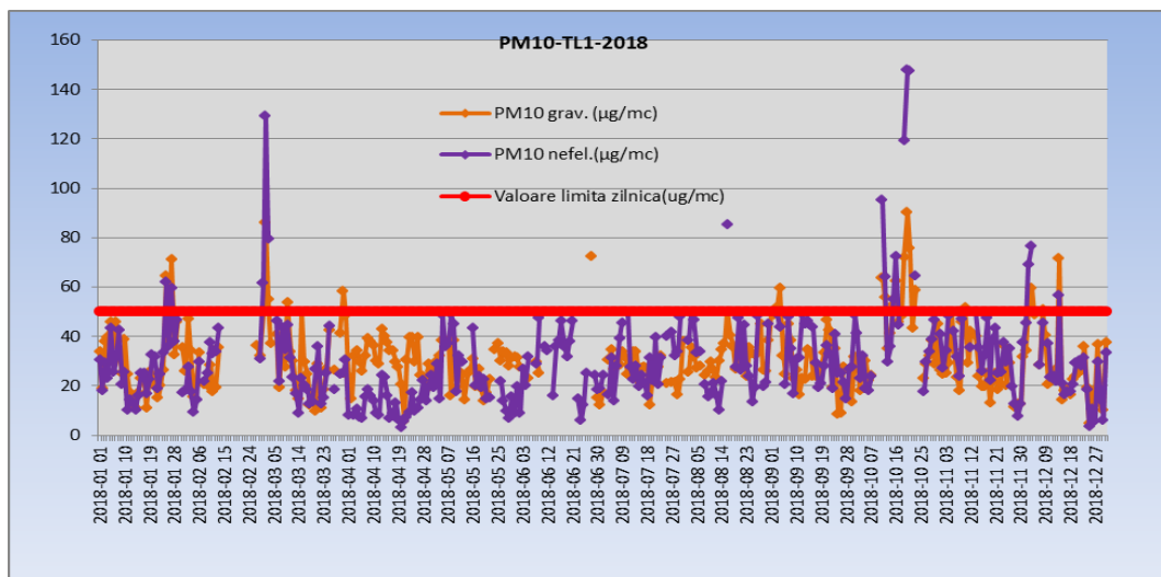
Fig.12 TL1: Concentrații medii zilnice PM10 grav. - 2018
