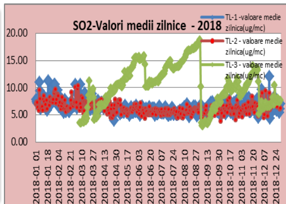
Fig. 4 Concentrații medii zilnice SO2 -2018
