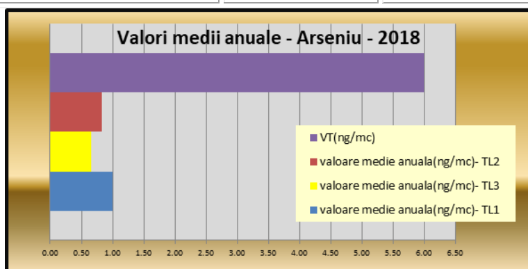
Figura nr.17 Valori medii anuale – arseniu – 2018
