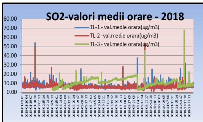
Fig. 3 Concentrații medii orare SO2 -2018
