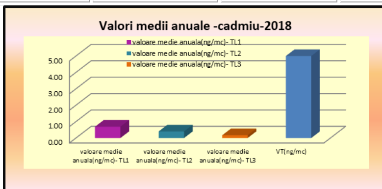
Figura nr.18 Valori medii anuale – cadmiu – 2018
