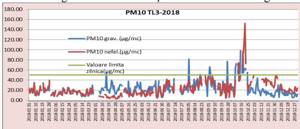
Fig.14 TL3:Concentrații medii zilnice PM10 grav.-2018
