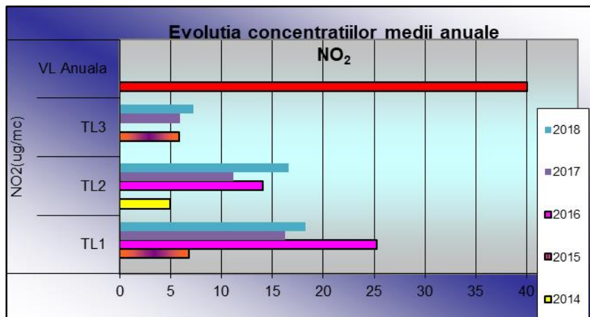
Fig. 2 Valorile concentrației medii anuale de \text{NO}_2
