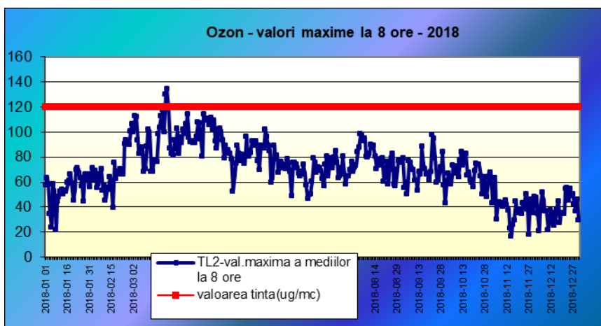
Fig. 7 Valori maxime zilnice a mediilor la 8 ore – O3 – 2018
