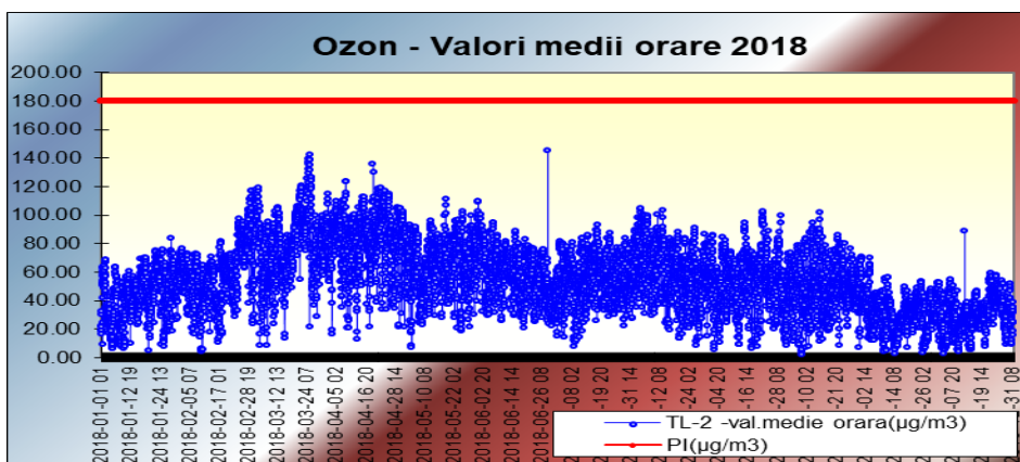
Fig. 6. Concentrații medii orare O3-2018
