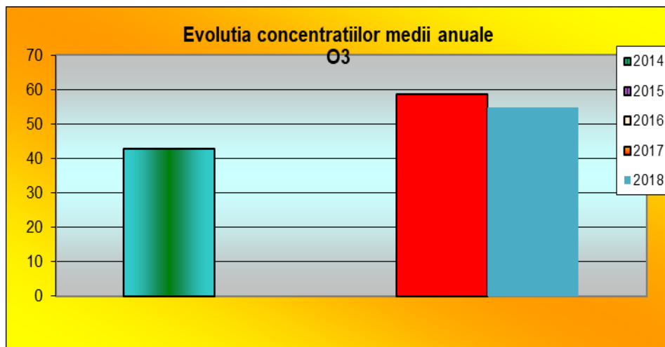
Fig. 8 Valorile concentrației medii anuale de O 3
