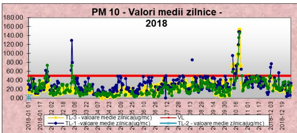
Fig.11 Concentrații medii zilnice PM10 nefelometric -2018
