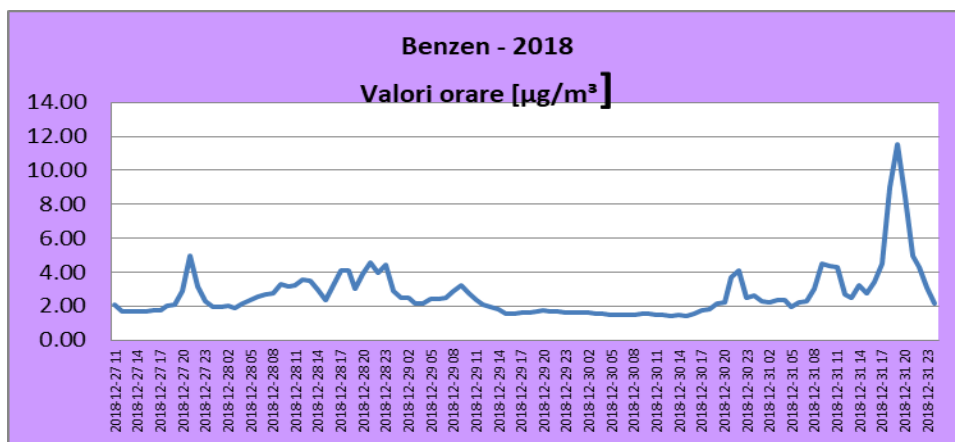
Concentrații medii orare benzen - 2018
