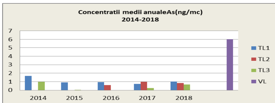
Fig.20 - Concentrații medii anuale As
