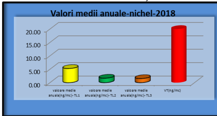
Figura nr.18 Valori medii anuale – nichel – 2018
