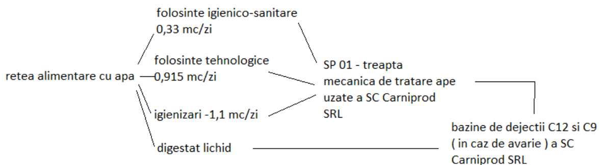
Fig. 2 Procesul apei menajere si a apei pentru spalare
