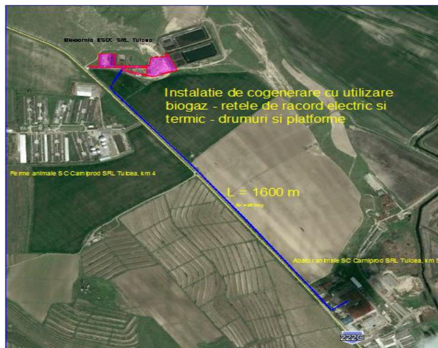
Fig. 1- pozitionare amplasament instalatie de cogenerare cu biogaz –retele racord electric si termic – drumuri si platforme
