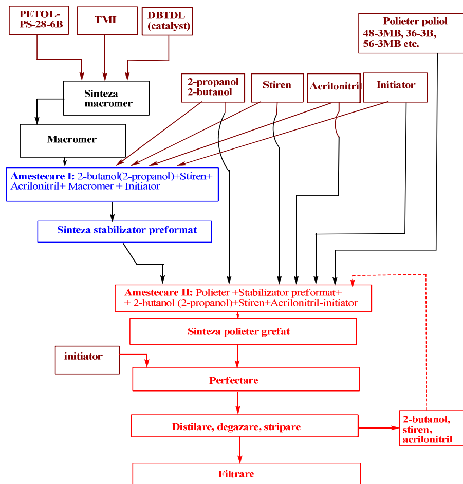
SCHEMA IV. Fluxuri tehnologice pentru sinteza macromerului (în negru), stabilizatorului preformat (în albastru) și a polieterului grefat (în roșu). Materii prime (în maro)
