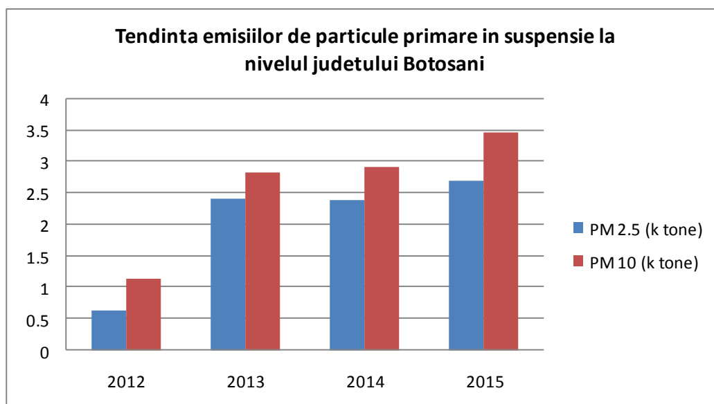
Figura I.3.1.12. Tendința emisiilor de particule primare în suspensie la nivelul județului Botoșani
