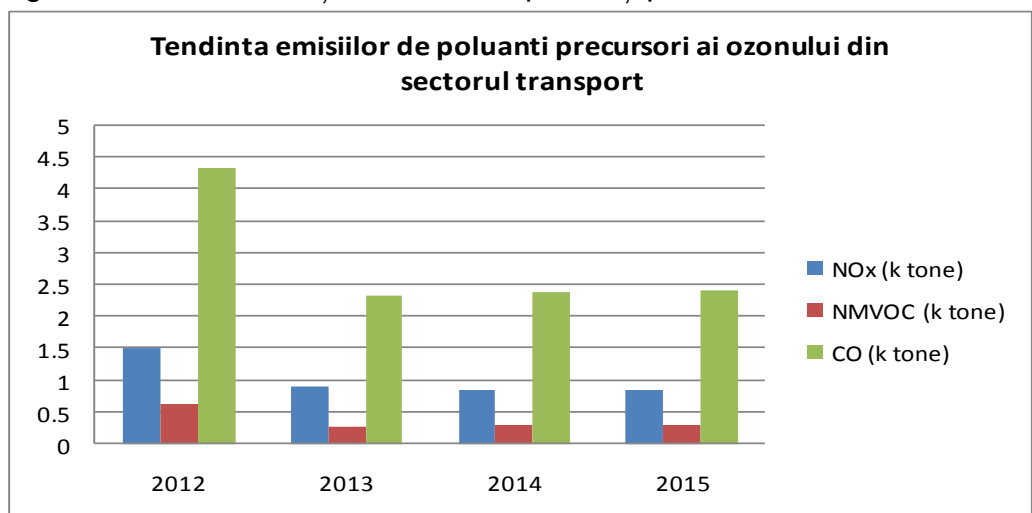
Figura I.3.1.10. Tendința emisiilor de poluanți precursori ai ozonului din sectorul transport
