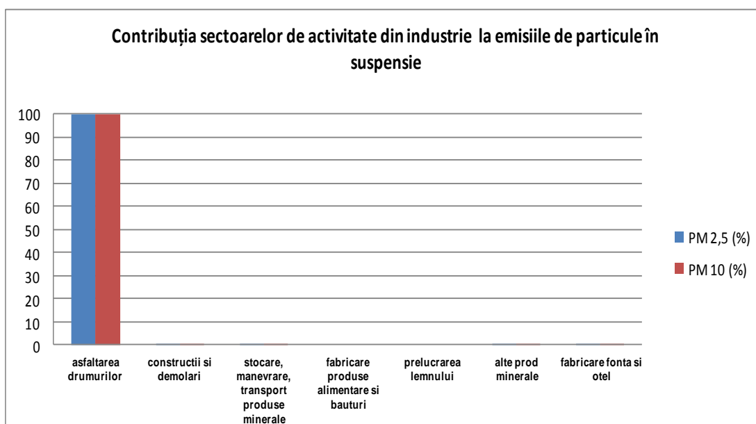
Figura I.2.1.2.5. Contribuția sectoarelor de activitate din industrie la emisiile de particule în suspensie
