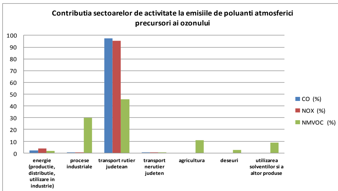
Figura I.2.1.2.2. Contribuția sectoarelor de activitate la emisiile de poluanți atmosferici precursori ai ozonului
