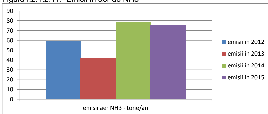
Figura I.2.1.2.11. Emisii în aer de NH3
