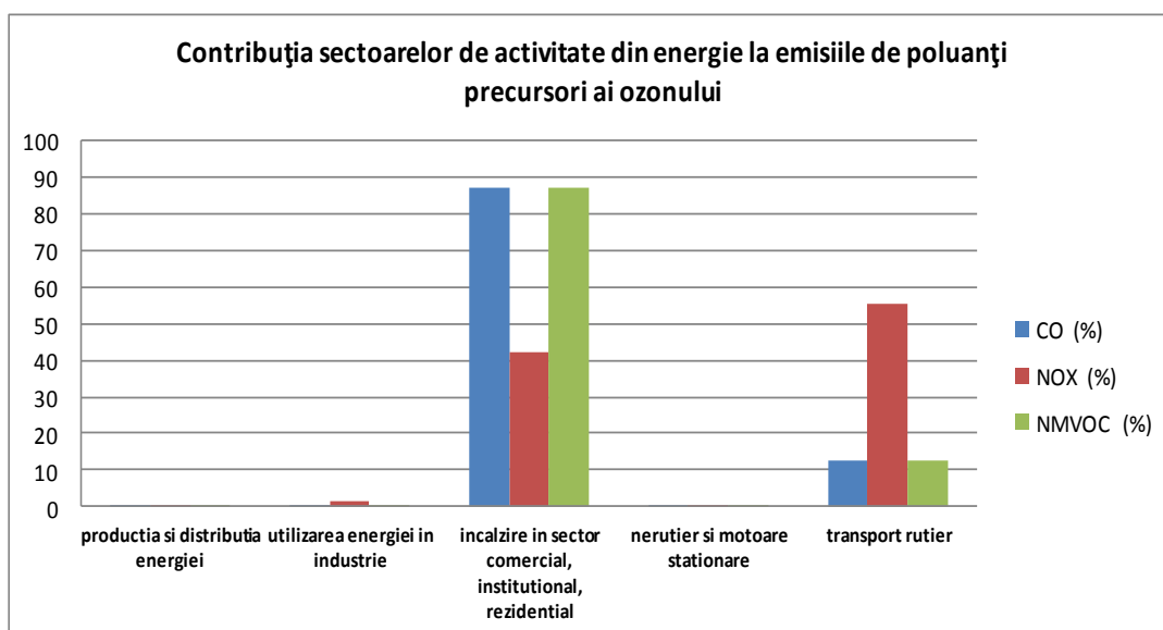
Figura I.2.1.1.2. Contribuția sectoarelor de activitate din energie la emisiile de poluanți precursori ai ozonului
