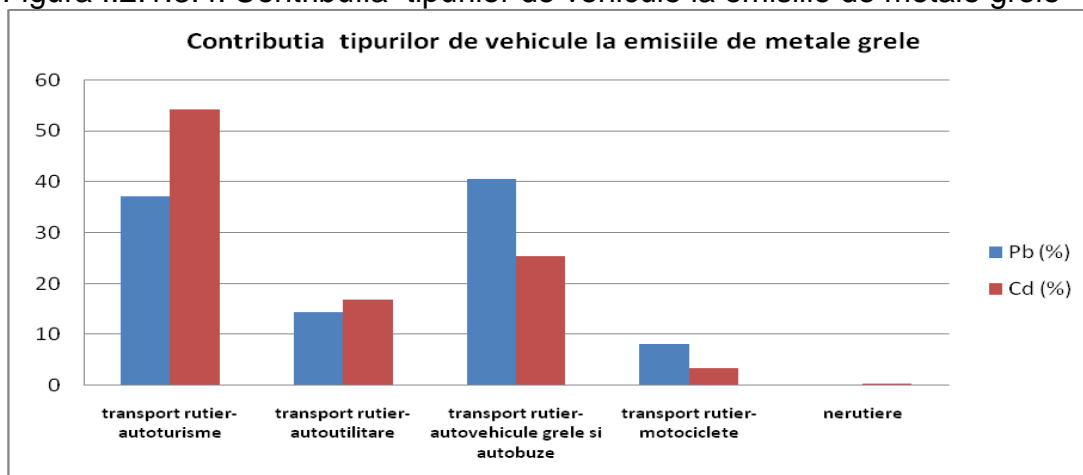
Figura I.2.1.3.4. Contribuția tipurilor de vehicule la emisiile de metale grele
