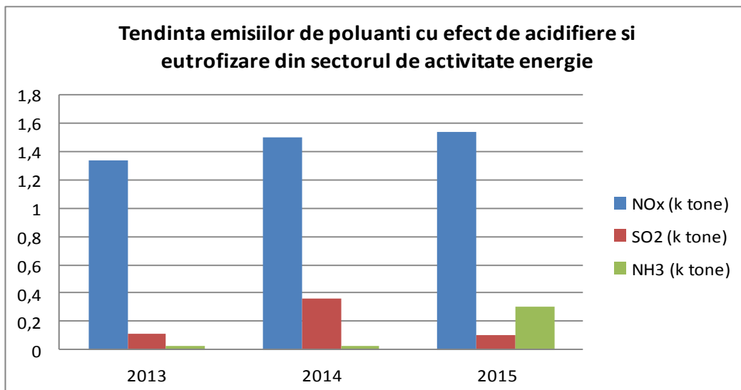
Figura I.3.1.2. Tendința emisiilor de poluanți cu efect de acidifiere și eutrofizare din sectorul de activitate energie
