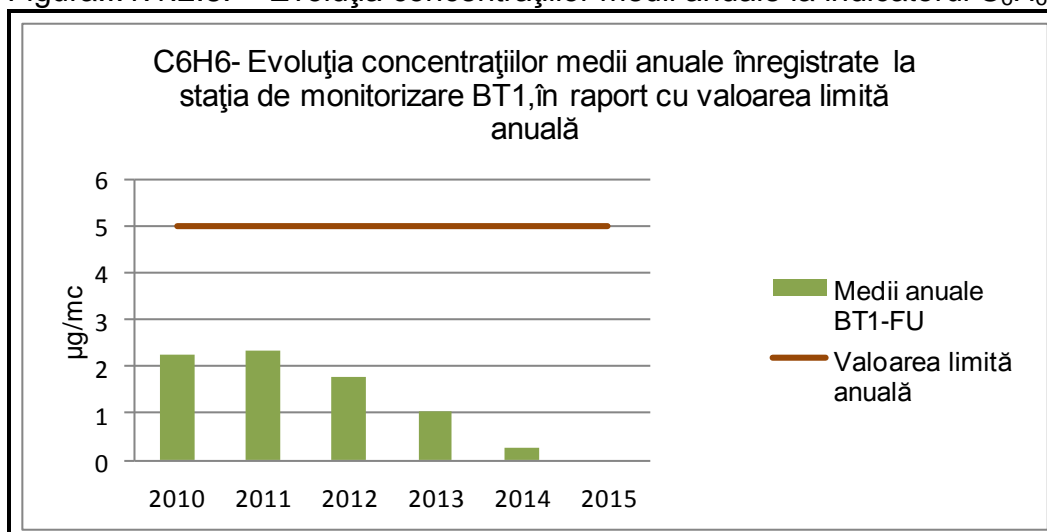
Figura:I.1.1.2.8. - Evoluția concentrațiilor medii anuale la indicatorul C 6 H 6
