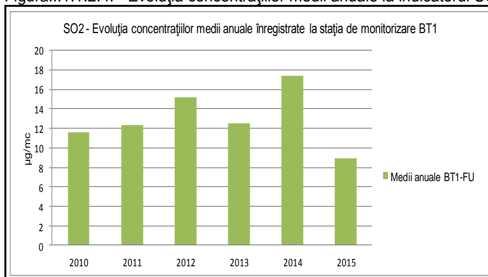
Figura:I.1.1.2.4. - Evoluția concentrațiilor medii anuale la indicatorul SO2
