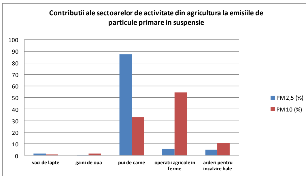
Figura I.2.1.4.3. Contributii ale sectoarelor de activitate din agricultura la emisiile de particule primare in suspensie
