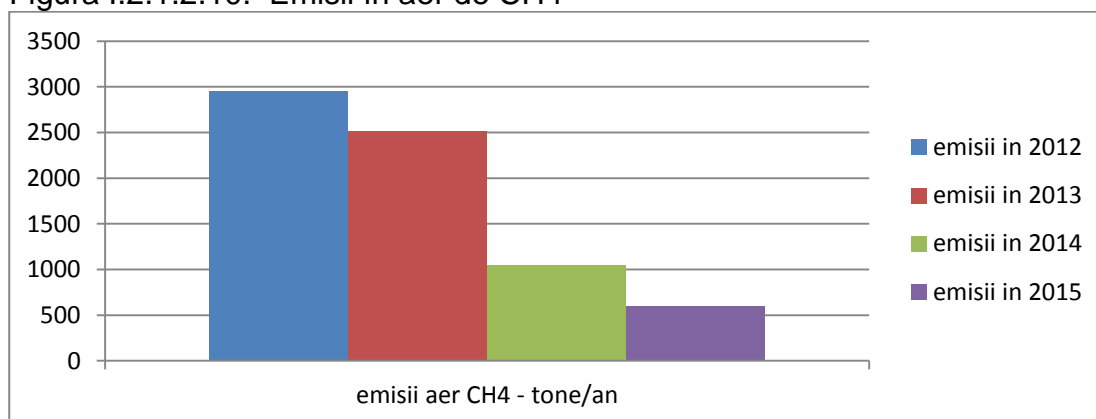
Figura I.2.1.2.10. Emisii în aer de CH4
