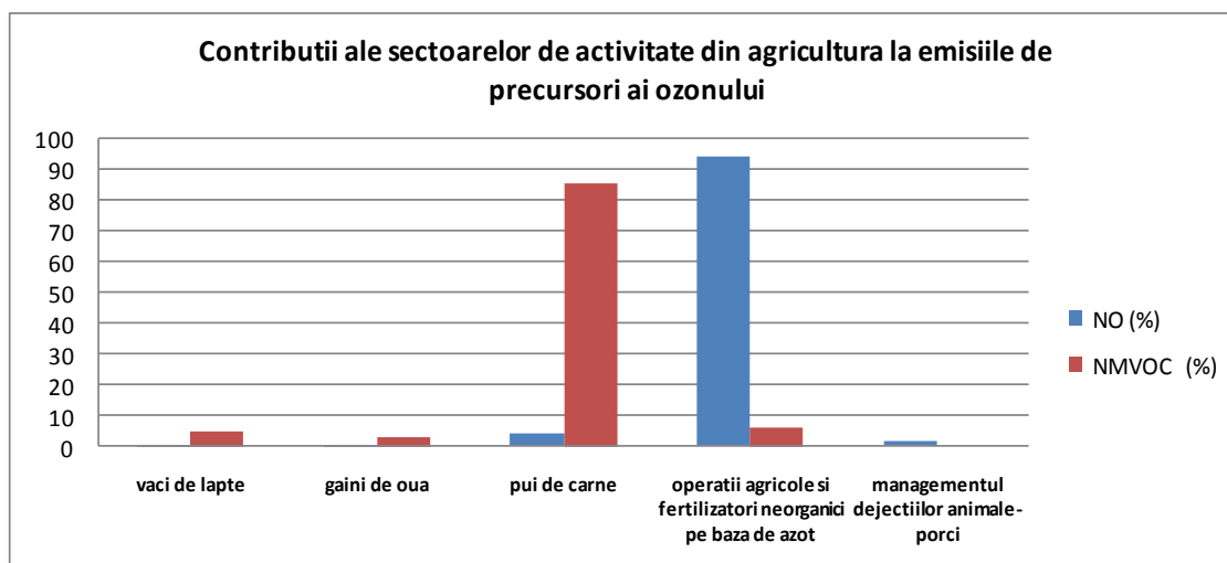
Fig.I.2.1.4.2.Contribuții ale sectoarelor de activitate din agricultură la emisiile de precursori ai ozonului
