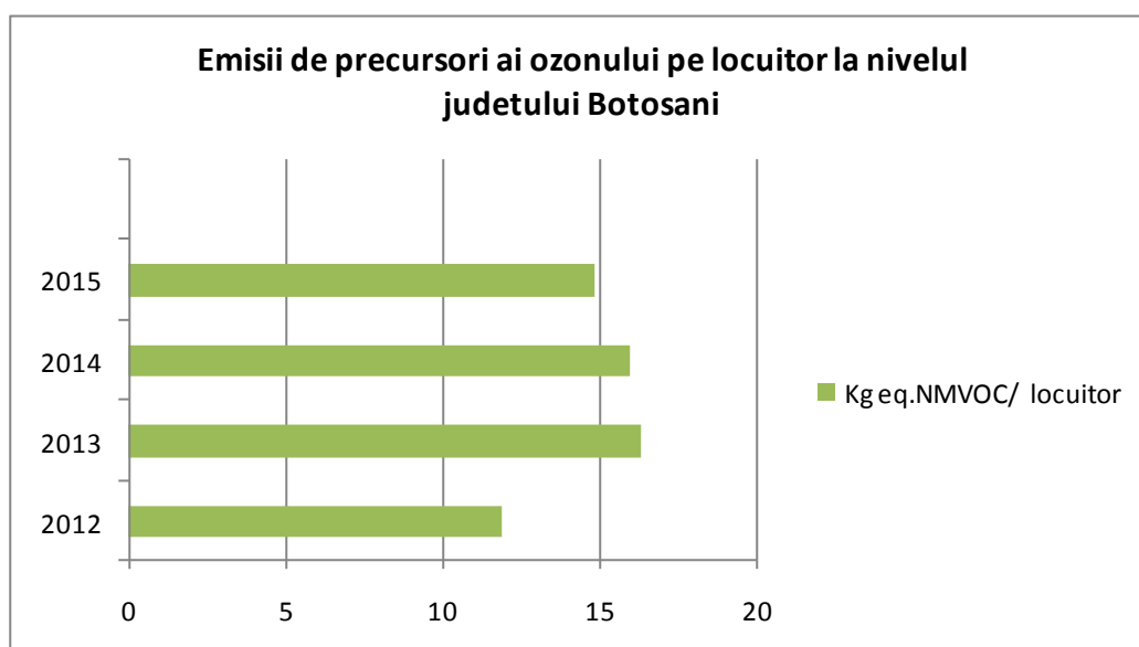
Figura I.3.1.7. Emisii de precursori ai ozonului pe locuitor la nivelul județului Botoșani
