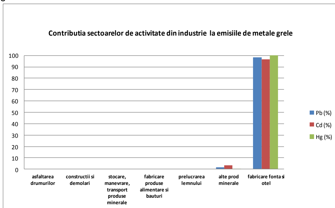
Figura I.2.1.2.7. Contribuția sectoarelor de activitate din industrie la emisiile de metale grele
