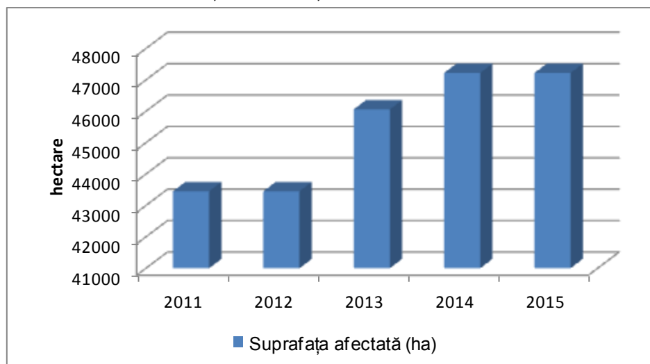
Figura III.2.1.1 Evoluția suprafețelor afectate de alunecări de teren
