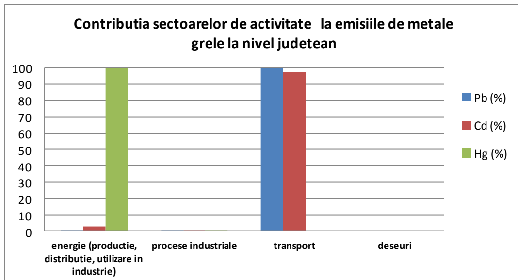
Figura I.2.1.2.6. Contribuția sectoarelor de activitate la emisiile de metale grele la nivel județean
