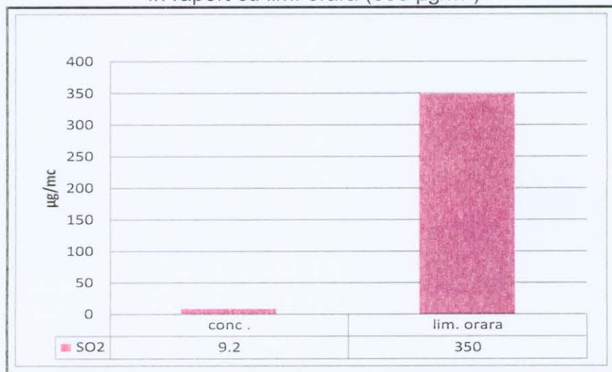
Fig. 3.1.1. Concentrația medie orară de SO 2 , în raport cu lim. orară (350 \mu\text{g}/\text{m}^3 )
