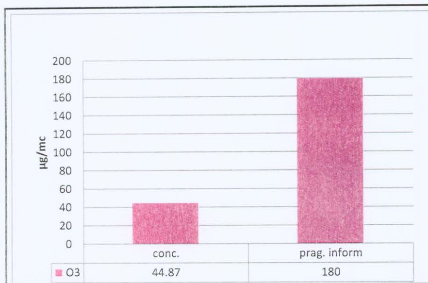
Fig. 3.4.1. Concentrația medie anuală de O 3 , în raport cu val.pragului de informare (180μg/m 3 )
