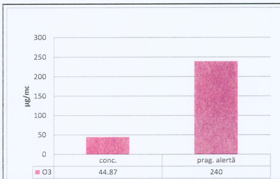
Fig. 3.4.2. Concentrația medie anuală de O 3 , în raport cu val.pragului de alertă (240μg/m 3 )
