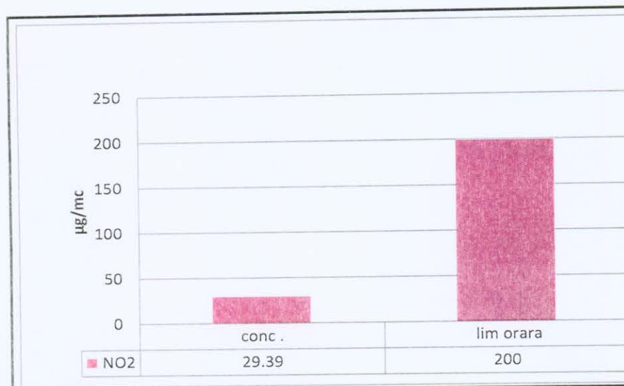
Fig. 3.2.1. Concentrația medie orară de NO 2 , în raport cu lim. orară (200 μg/m 3 )
