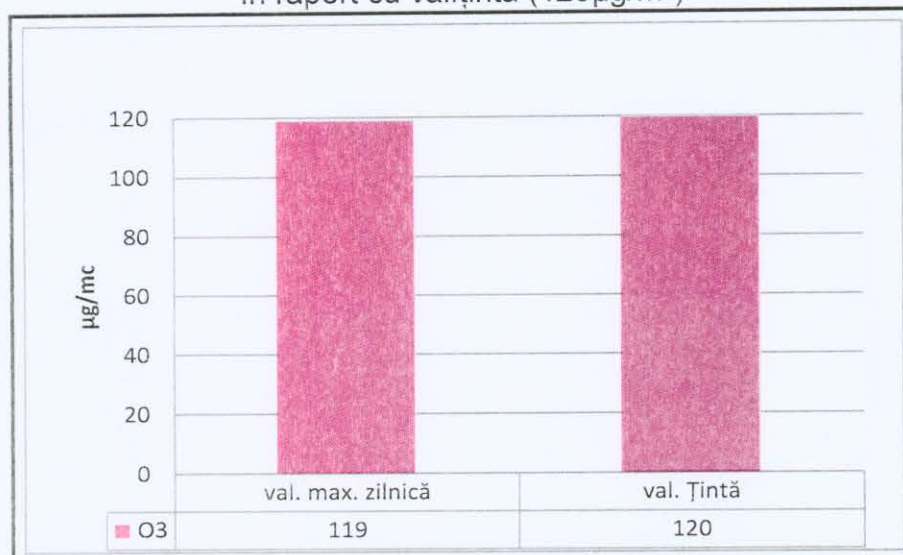
Fig. 3.4.2. Valoarea maximă zilnică de O 3 , în raport cu val. țintă (120 μg/m 3 )
