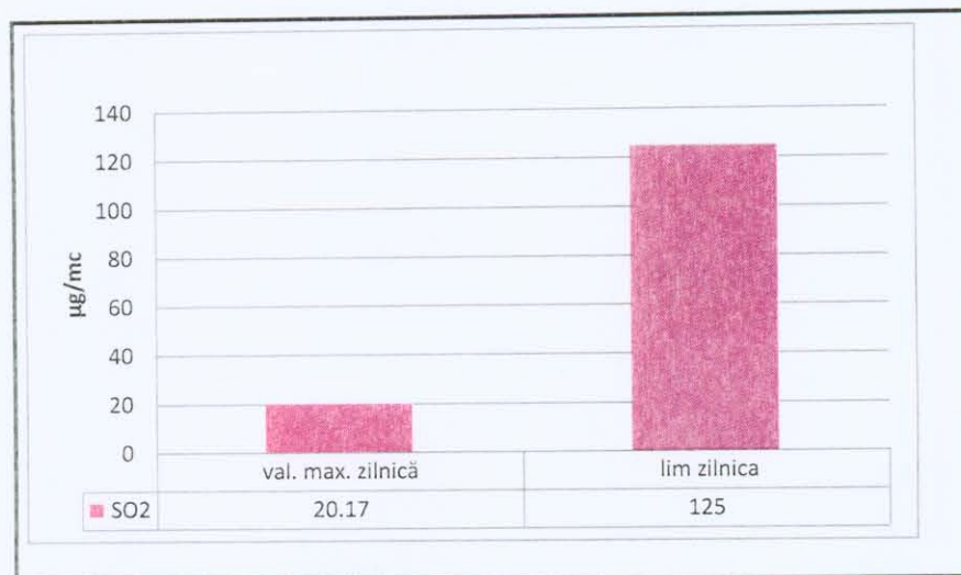
Fig. 3.1.2. Valoarea maximă zilnică de \text{SO}_2 , în raport cu lim. zilnică ( 125 \mu\text{g}/\text{m}^3 )
