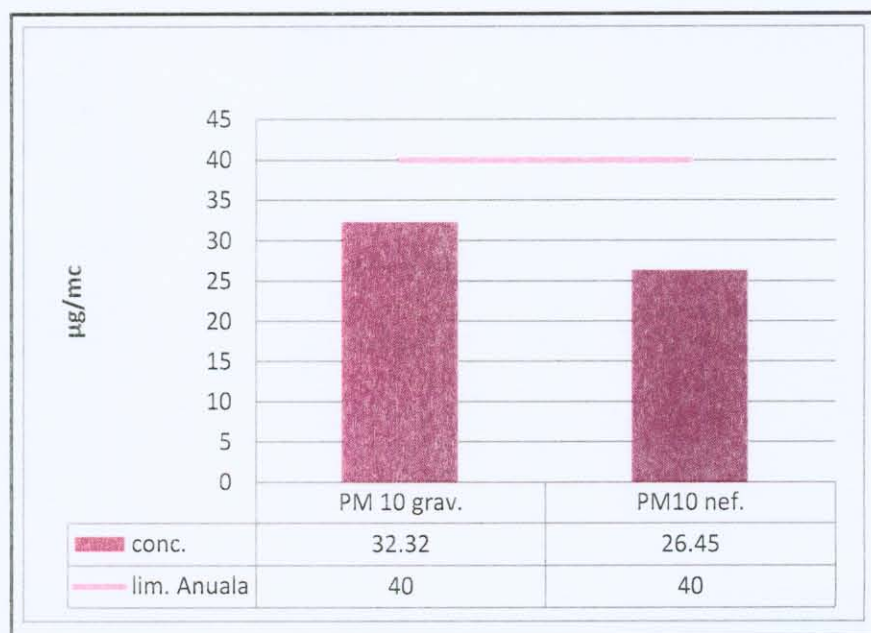
Fig. 3.6.1.1. Concentrația medie anuală de PM10 , în raport cu val. lim. anuală (40 \mu\text{g}/\text{m}^3 )
