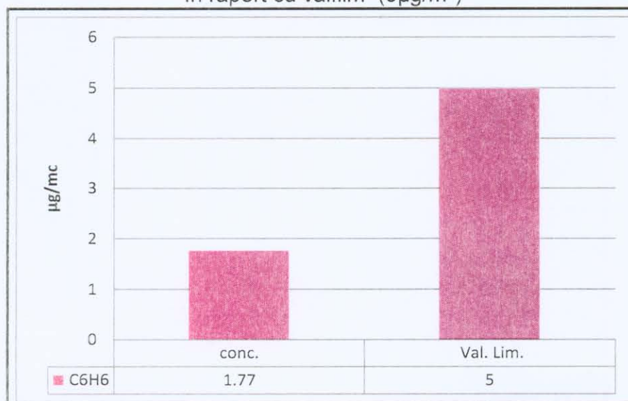
Fig. 3.5.1. Concentrația medie anuală la C 6 H 6 , în raport cu val.lim (5 μg/m 3 )
