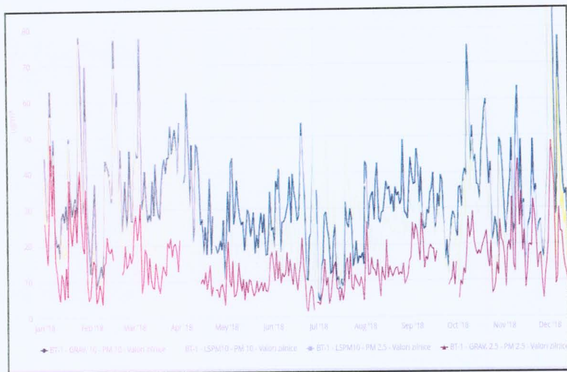
Fig. 3.6.1.4.Evoluția indic. PM10 și PM2,5.
