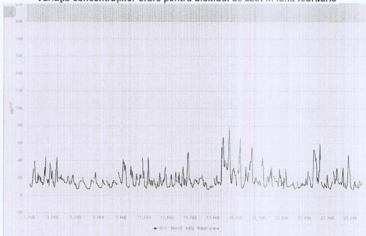
Variația concentrațiilor orare pentru dioxidul de azot în luna februarie
