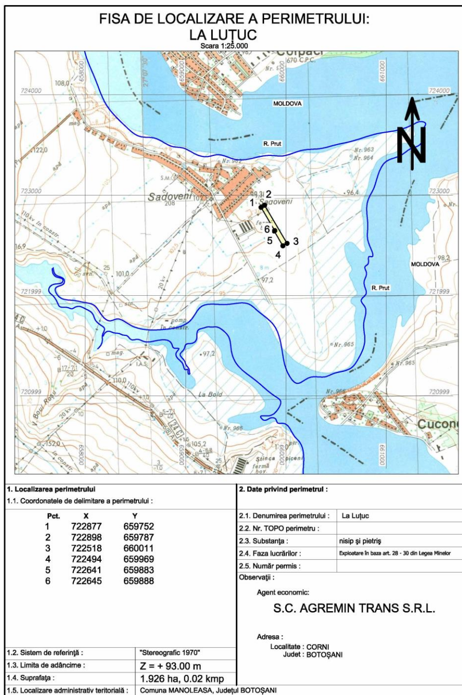
Figura 3. Fisa perimetrului
