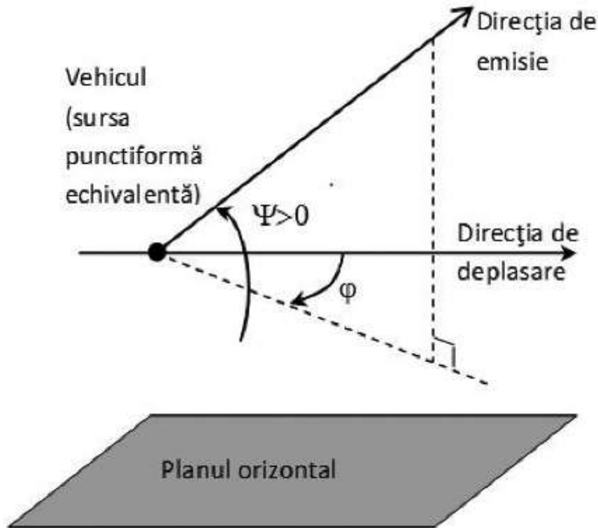
Figura [2.3.b]: Definierea geometrică
