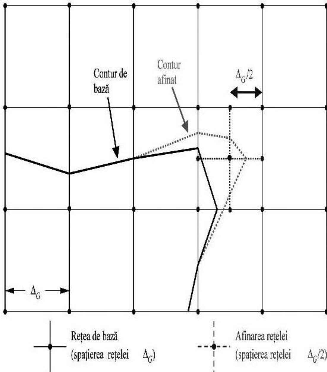
Figura 2.7.s: Rețeaua standard și afinarea rețelei
