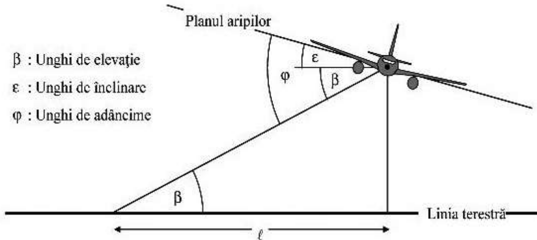
Figura 2.7.m: Unghiurile dintre observator și aeronavă în plan perpendicular pe traiectoria de zbor
