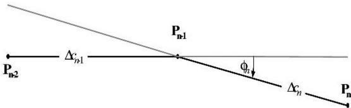
Figura 2.7.v: Parametrii geometrici care definesc condițiile algoritmului de trasare Anumite constrângeri trebuie să fie impuse pentru a garanta estimarea curbei cu un grad satisfăcător de precizie (a se vedea figura 2.7.v)
