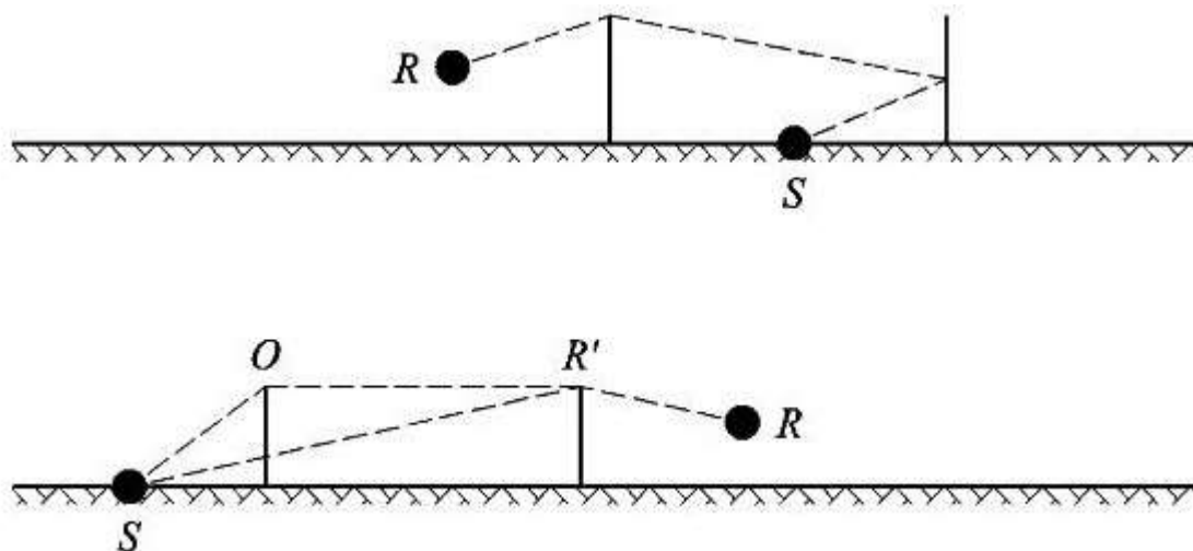
Figura 2.5.j: Diferența traiectoriei în prezența unei difracții: secțiunea transversală actuală (partea superioară), secțiunea transversală nedeschisă (partea inferioară)
