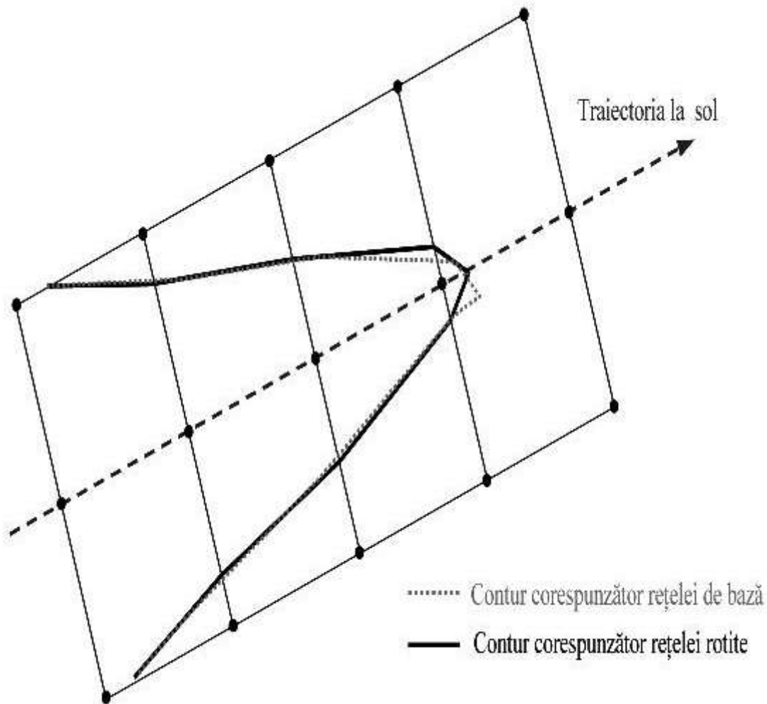
Figura 2.7.t: Utilizarea unei rețele rotite
