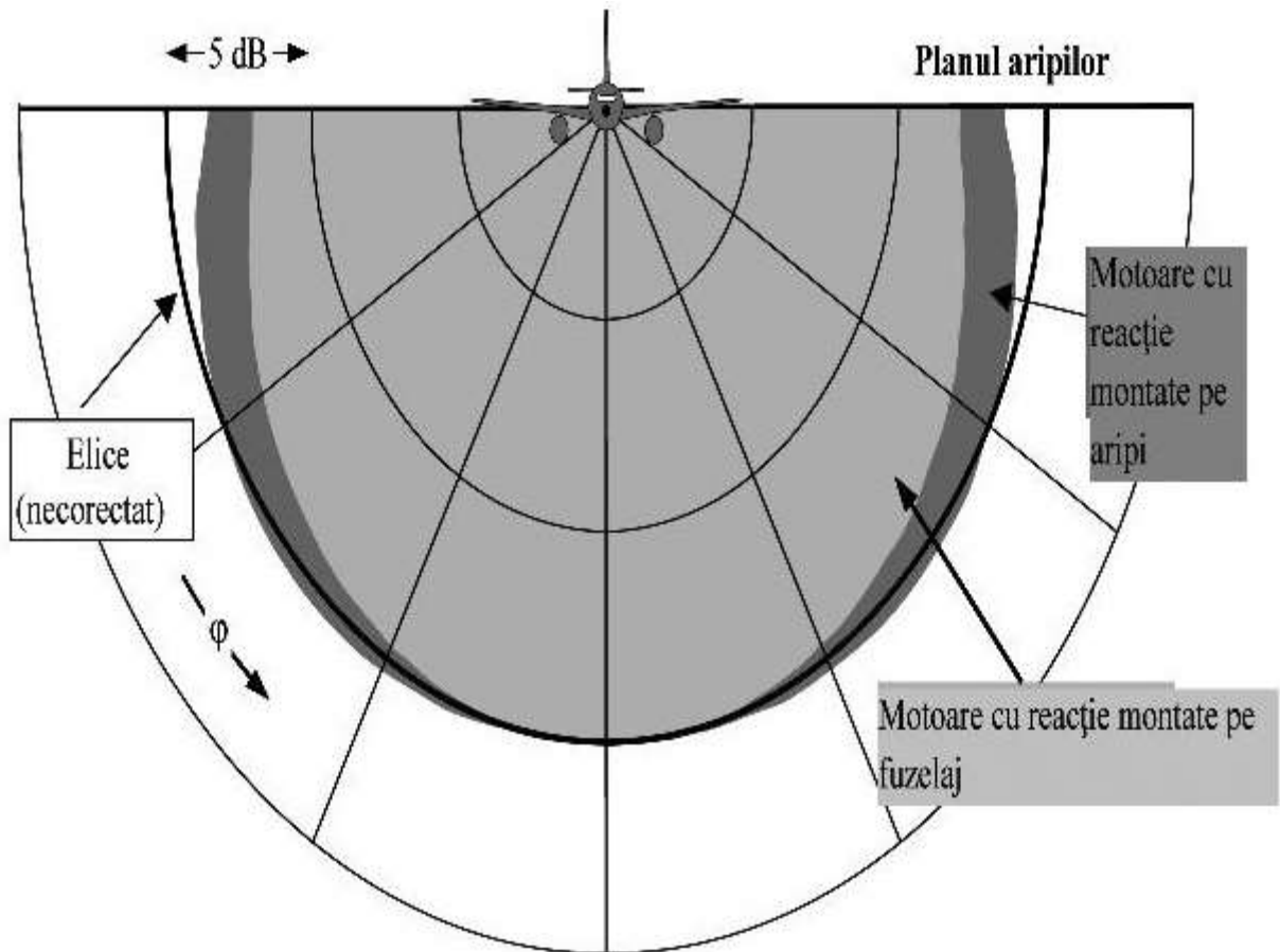
Figura 2.7.n: Direcivitatea laterală a efectelor amplasării
