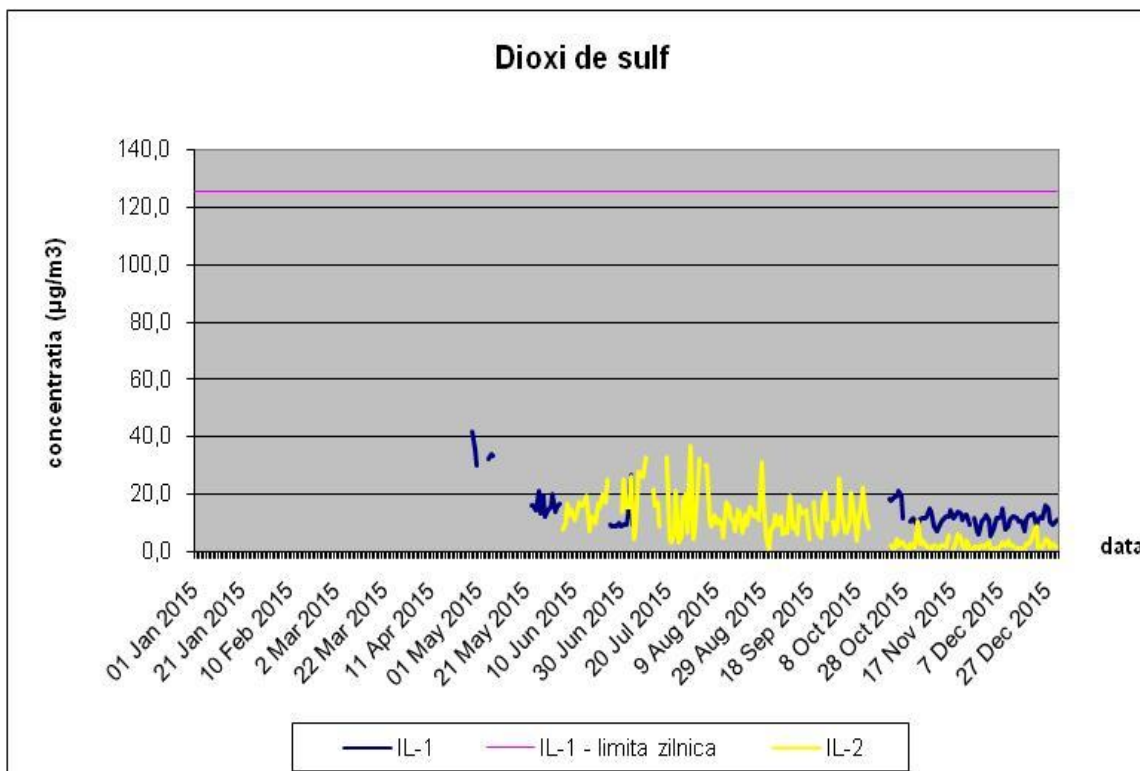
Fig. 1.6 Graficul concentrațiilor medii zilnice de dioxid de sulf
