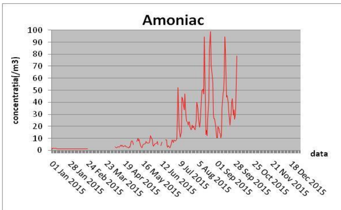
Fig. 1.20 Graficul concentrațiilor medii zilnice de amoniac
