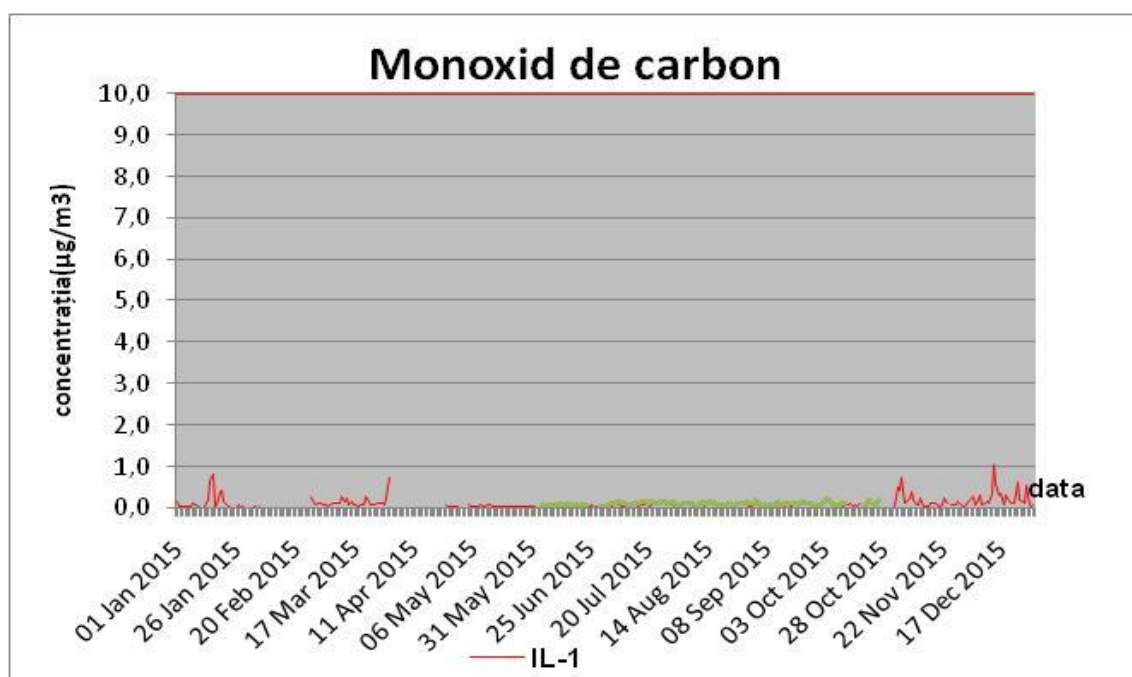
Fig. 1.17 Graficul concentrațiilor medii orare - monoxid de carbon
