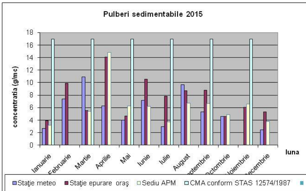
Fig. 1.14 Reprezentarea grafică a cantităților de pulberi sedimentabile în municipiul Slobozia în anul 2015
