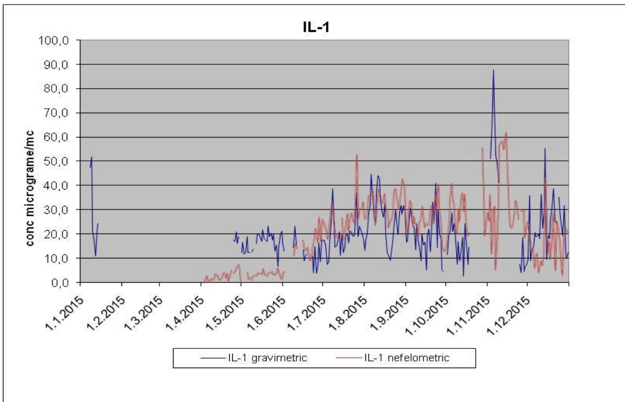
Fig. 1.11 Grafic comparativ pulberi în suspensie PM10 nefelometric-gravimetric stația IL-1 și stația IL-2
