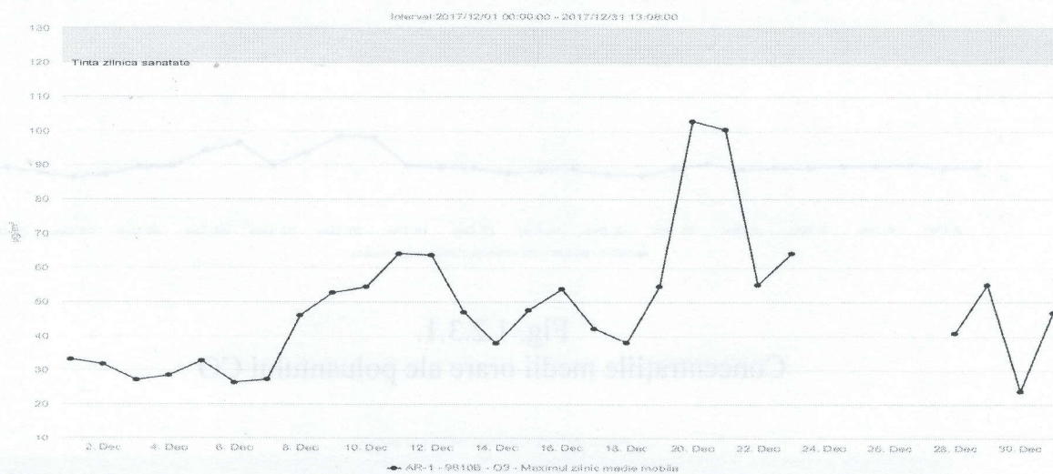
Fig. 1.2.4.1. Concentrațiile medii orare ale poluantului \text{O}_3
