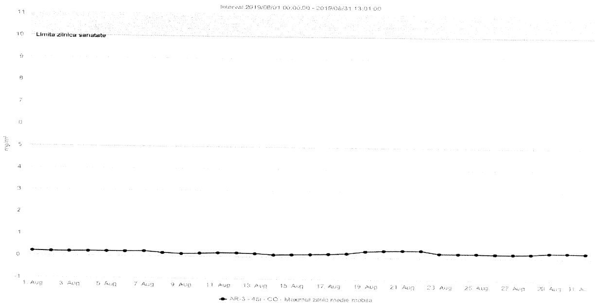
Fig. 1.2.3.3. Concentrațiile medii orare ale poluantului CO
