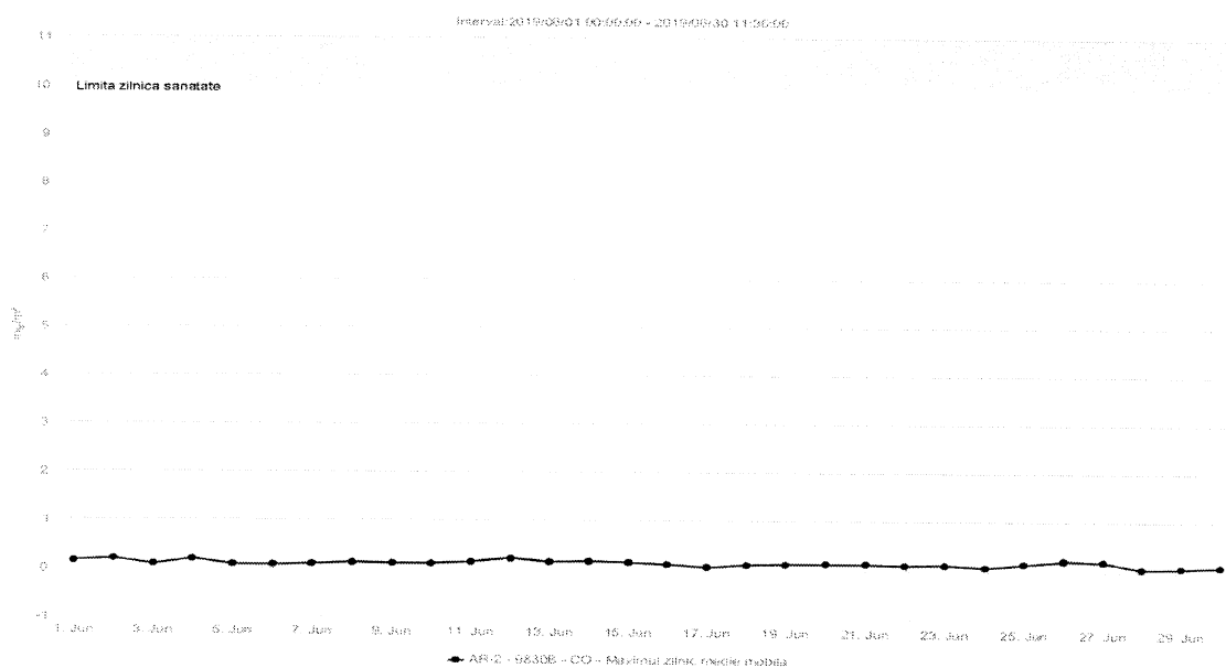
Fig. 1.2.3.2. Concentrațiile medii orare ale poluantului CO
