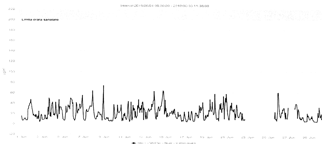
Fig.1.2.2.1. Concentrațiile medii orare ale poluantului NO 2
