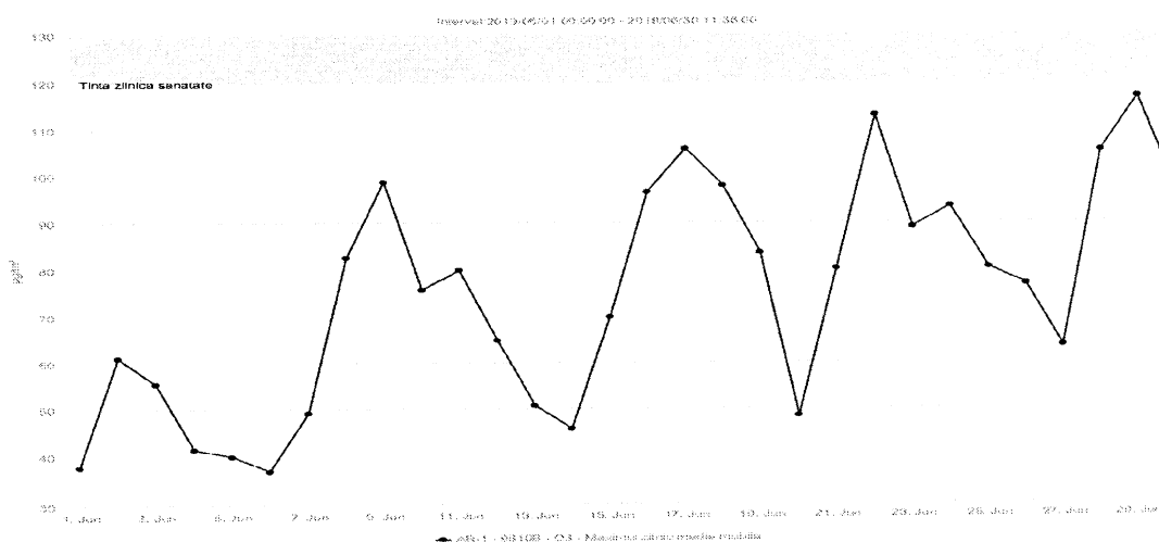
Fig. 1.2.4.1. Concentrațiile medii zilnice ale poluantului \text{O}_3
