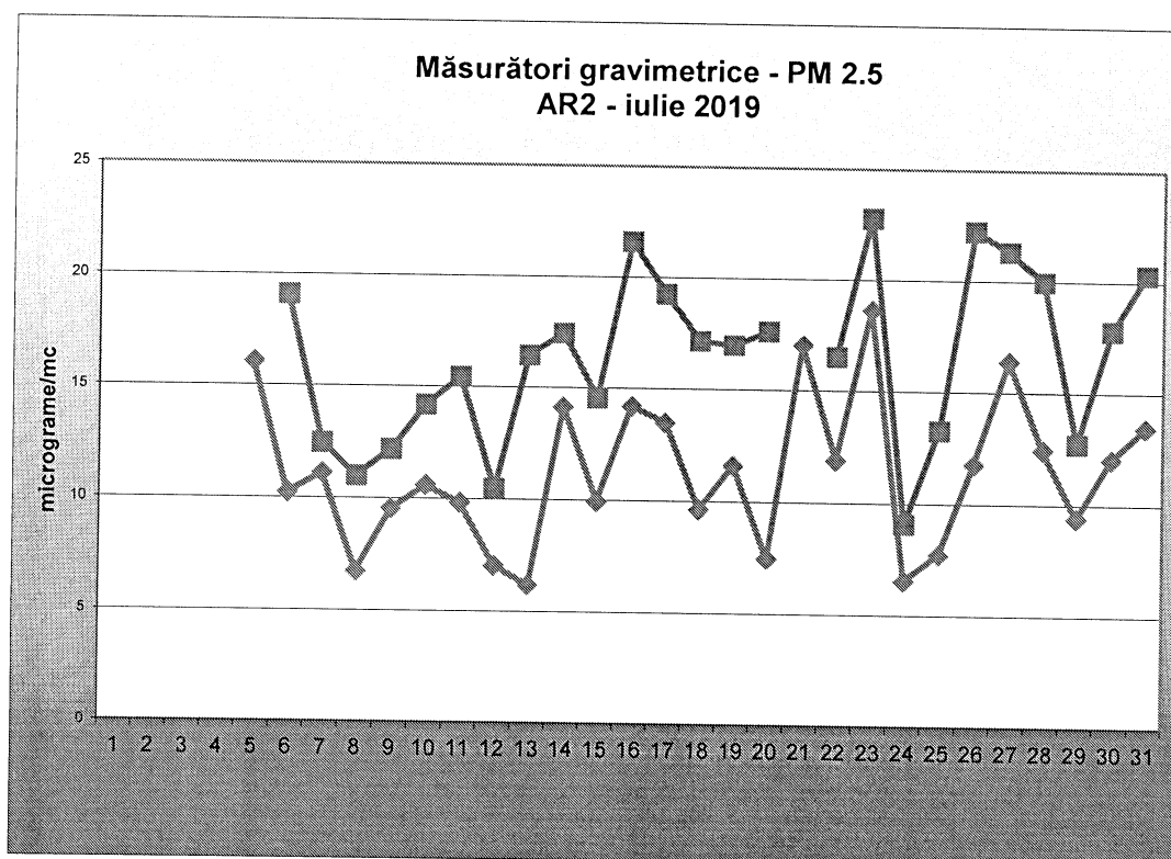
În fig.1.2.5.3. se prezintă grafic, evoluția măsurătorilor gravimetrice la PM2.5 la stația de monitorizare AR2
