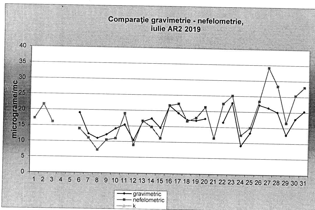
În fig.1.2.5.3. se prezintă grafic, evoluția măsurătorilor gravimetrice la PM2.5 la stația de monitorizare AR2
