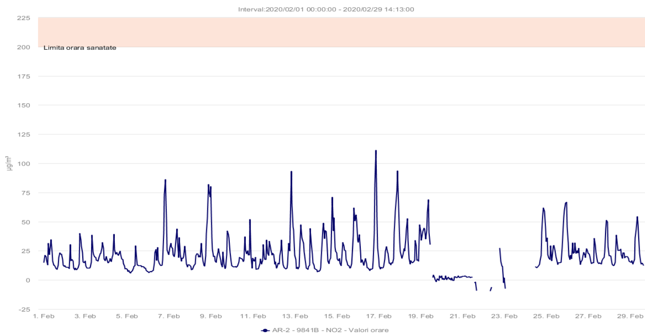
Fig.1.2.2.3. Concentrațiile medii orare ale poluantului NO 2
