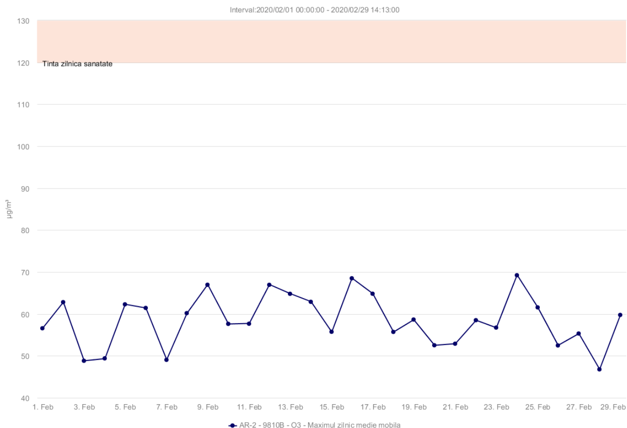
Fig. 1.2.4.2. Concentrațiile mediilor zilnice ale poluantului O 3
