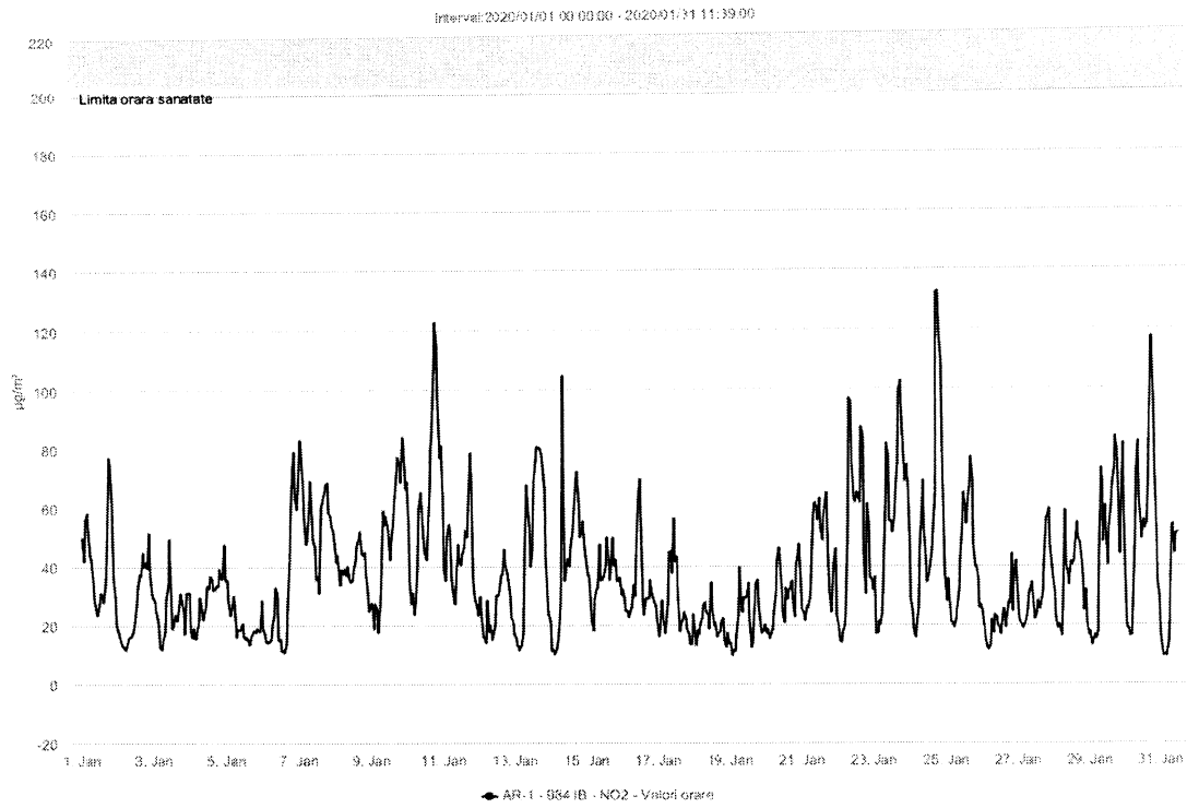
Fig.1.2.2.3. Concentrațiile medii orare ale poluantului NO 2
