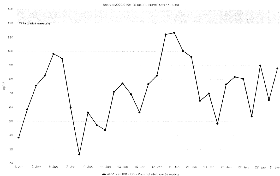
Fig. 1.2.4.1. Concentrațiile medii zilnice ale poluantului \text{O}_3
