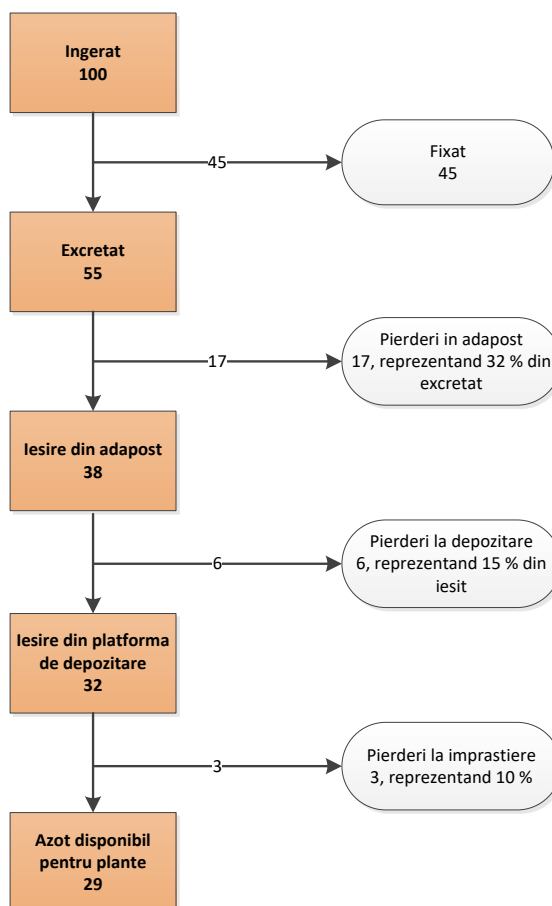
Diagrama fluxului de azot în cazul gestionării dejecțiilor de la puii crescuți la sol, pe așternut
