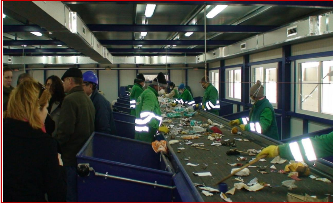
Figura VII.1.3.2.12. Incinta stației de sortare a deșeurilor reciclabile din cadrul depozitului Țuțora
