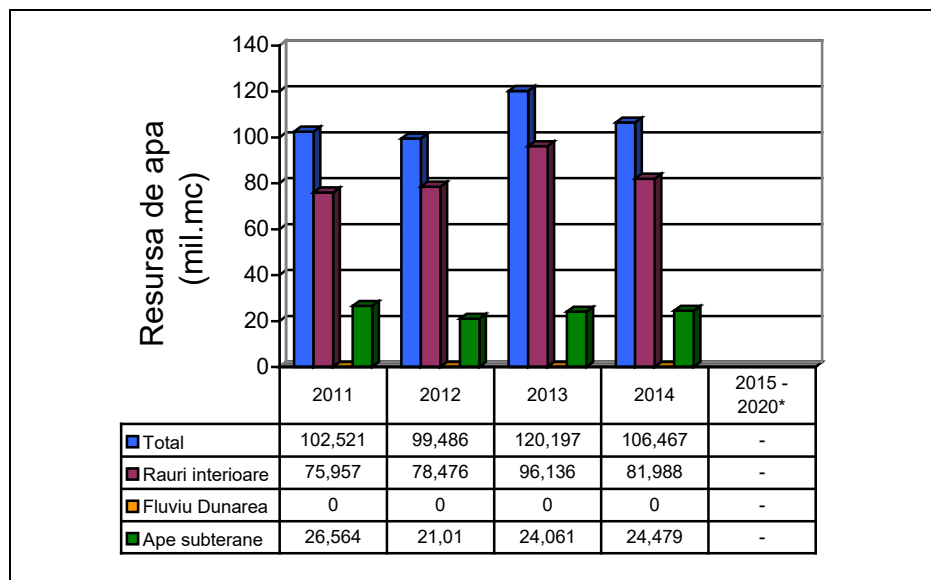
Figura II.1.1.1.1. Resursele de apă potențiale și tehnic utilizabile la nivel județului Iași, pe teritoriul administrat de S.G.A. Iași, în perioada anilor 2011-2020 (mil.mc)
