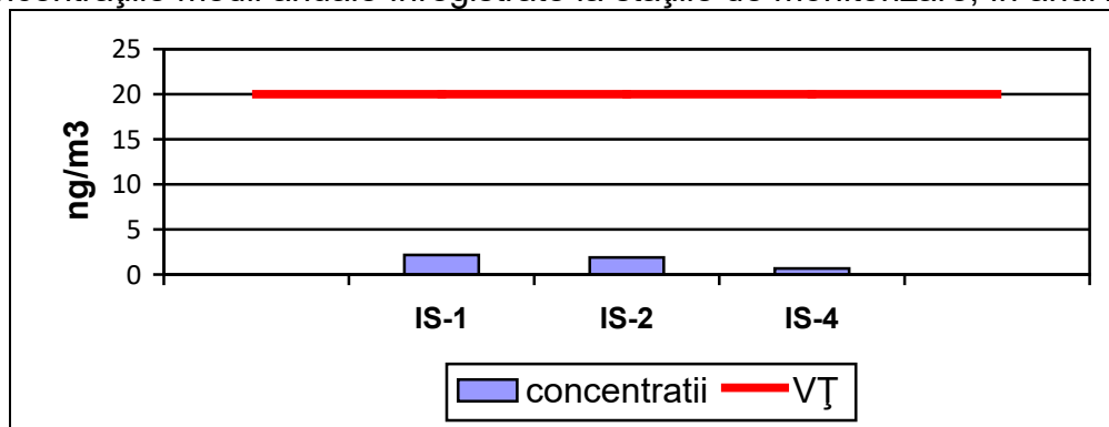
Figura I.1.1.1.7. Ni gravimetric determinat din fracția PM10 – Concentrațiile medii anuale înregistrate la stațiile de monitorizare, în anul 2020
