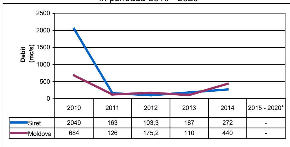
Figura II.1.1.3.7. Evoluția debitelor maxime înregistrate pe cursurile de apă Siret și Moldova, în perioada 2010 - 2020
