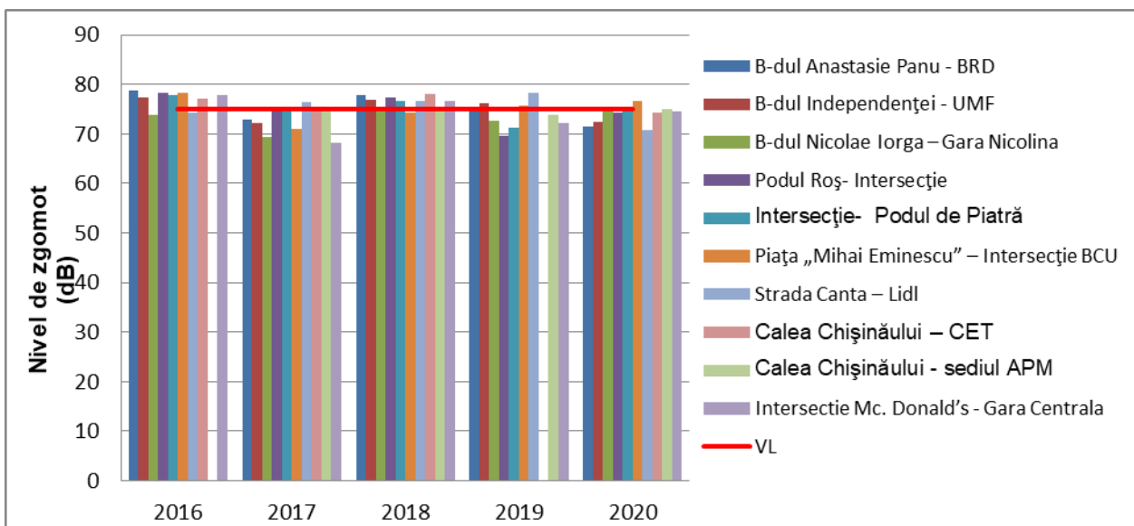
Figura VIII.1.2.1.12. Evoluția nivelului de zgomot echivalent maxim măsurat pe străzi de categoria tehnică I, magistrală, în perioada 2016 - 2020
