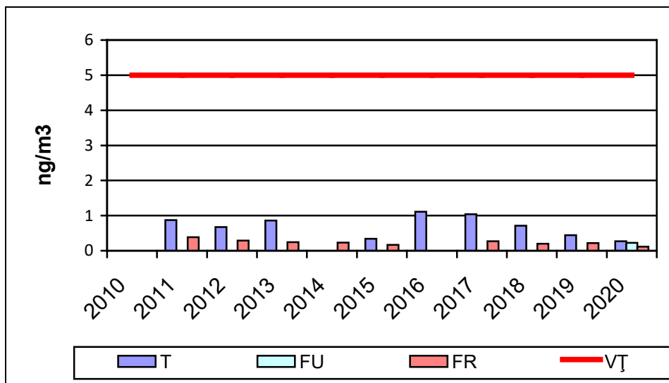
Figura I.1.1.2.7. Cd gravimetric determinat din fracția PM10 – Evoluția concentrațiilor medii anuale înregistrate la stațiile de monitorizare în raport cu VL anuală, în perioada 2010 – 2020
