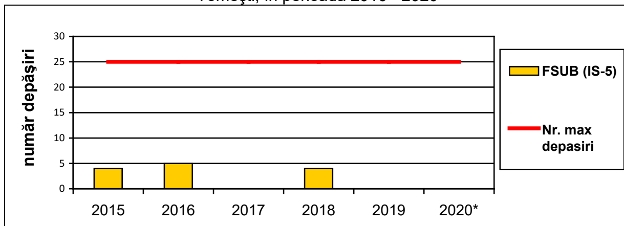
Figura VIII.1.1.1.2. Evoluția numărului de depășiri ale valorii țintă pentru ozon în IS-5 Tomești, în perioada 2016 - 2020
