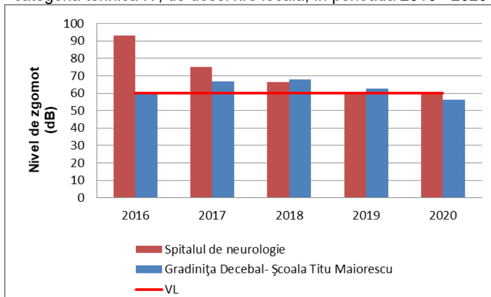
Figura VIII.1.2.1.15. Evoluția nivelului de zgomot echivalent maxim măsurat pe străzi de categoria tehnică IV, de deservire locală, în perioada 2016 - 2020
