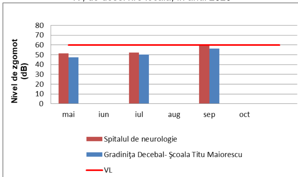
Figura VIII.1.2.1.5. Nivel de zgomot echivalent (dB) măsurat pe străzi de categoria tehnică IV, de deservire locală, în anul 2020
