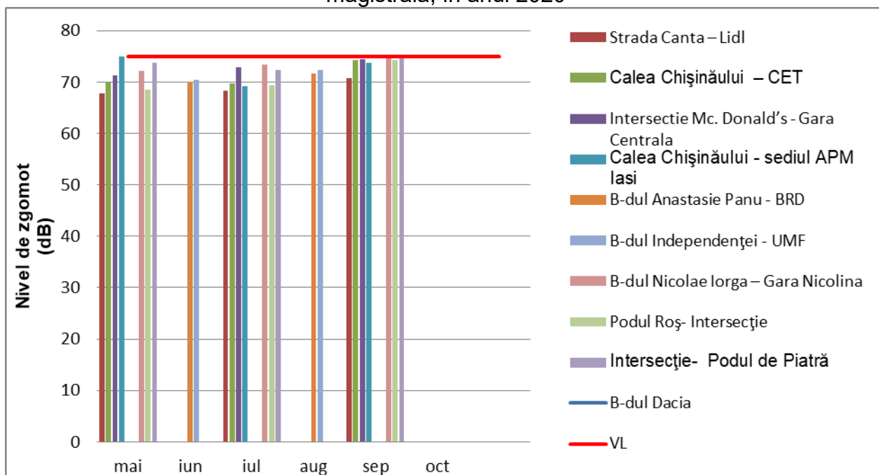
Figura VIII.1.2.1.2. Nivel de zgomot echivalent (dB) măsurat pe străzi de categoria tehnică I, magistrală, în anul 2020
