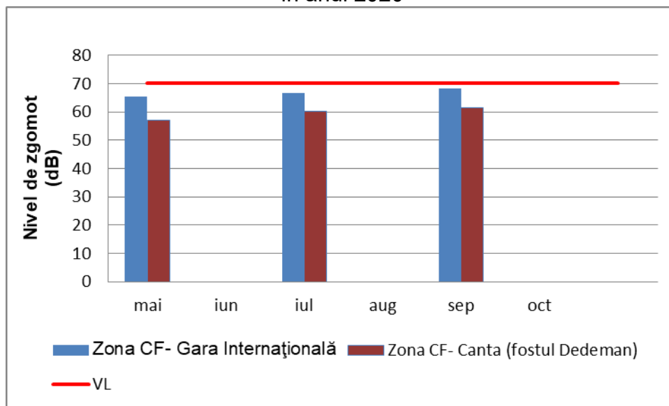
Figura VIII.1.2.1.8. Nivel de zgomot echivalent (dB) măsurat în zone feroviare, în anul 2020
