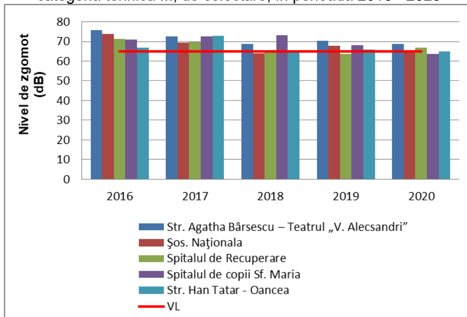
Figura VIII.1.2.1.14. Evoluția nivelului de zgomot echivalent maxim măsurat pe străzi de categoria tehnică III, de colectare, în perioada 2016 - 2020
