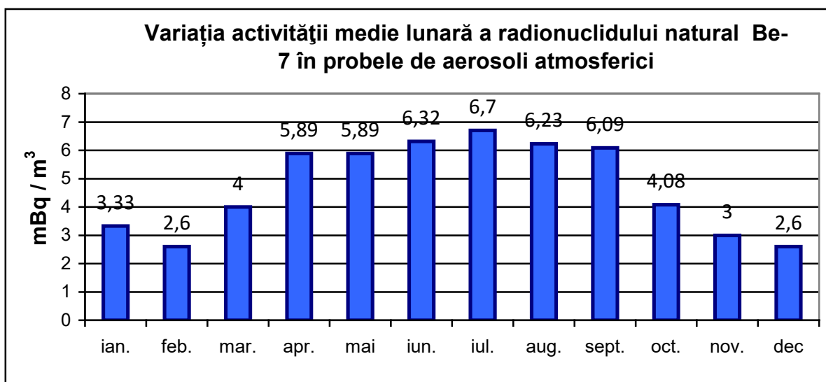
Figura IX.1.1.6. Variația activității medii lunare a radionuclidului natural Be-7 în probe de aerosoli atmosferici
