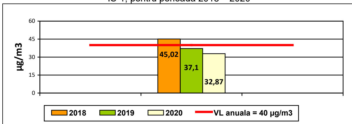
Figura I.1.1.3.2. Evoluția concentrației medii anuale pentru PM10 înregistrată la stația IS-1, pentru perioada 2018 – 2020
