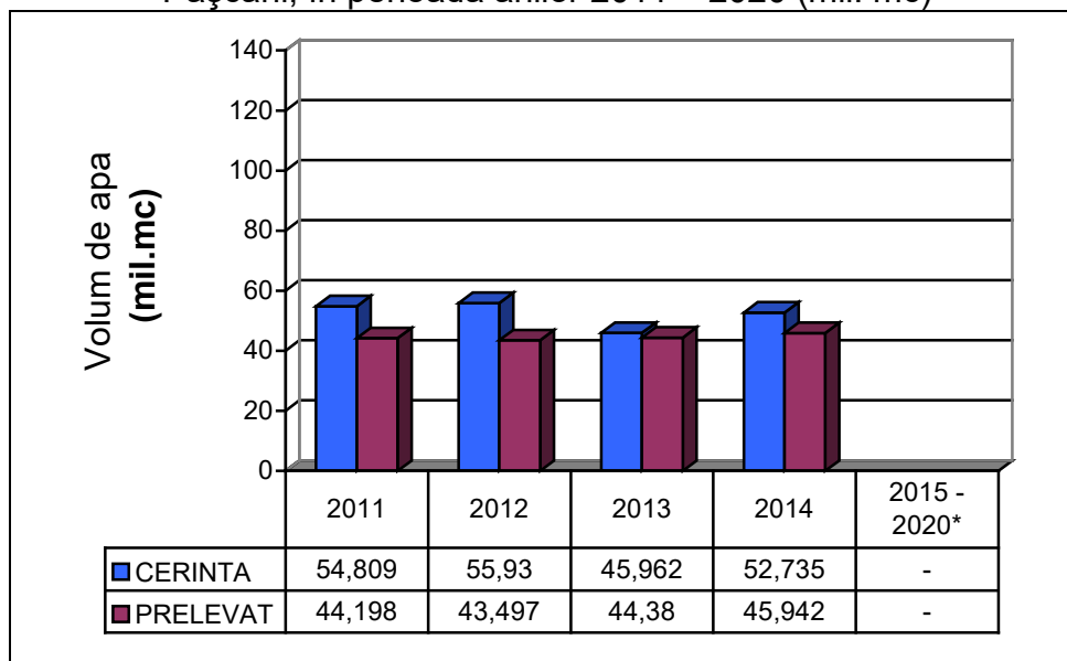
Figura II.1.1.2.2. Evoluția cerinței și prelevărilor de apă pe teritoriul administrat de S.H.I. Pașcani, în perioada anilor 2011 – 2020 (mil. mc)
