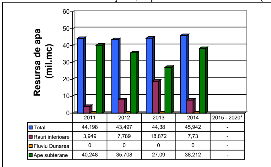
Figura II.1.1.1.2. Resursele de apă potențiale și tehnic utilizabile la nivel județului Iași, pe teritoriul administrat de S.H.I Pașcani, în perioada anilor 2011-2020 (mil.mc)
