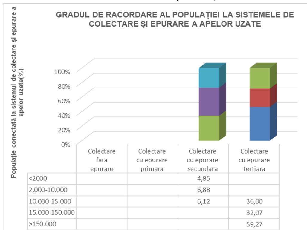
Figura II.2.2.2.1. Gradul de racordare al populației la sistemele de colectare și epurare a apelor uzate, diferențiat pe tipuri de aglomerări umane și niveluri de epurare, aflate în administrarea S.C. APAVITAL S.A. Iași; date specifice anului 2020
