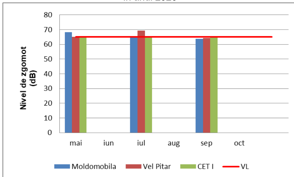
Figura VIII.1.2.1.9. Nivel de zgomot echivalent măsurat la limita incintelor industriale, în anul 2020
