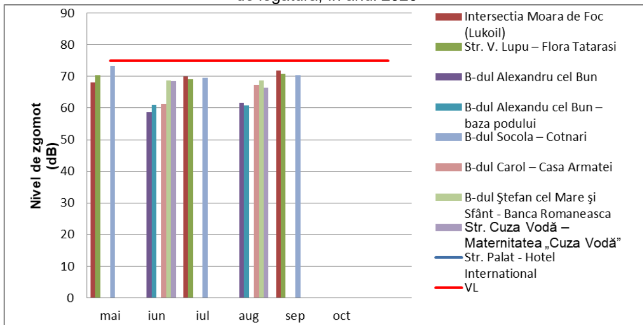
Figura VIII.1.2.1.3. Nivel de zgomot echivalent (dB) măsurat pe străzi de categoria tehnică II, de legătură, în anul 2020
