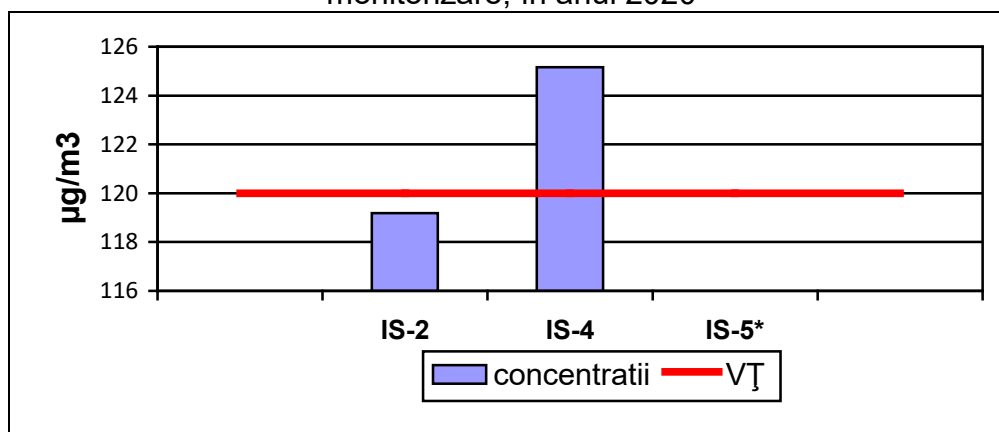
Figura I.1.1.1.8. Ozon – Maxima zilnică mediei pe 8 ore, înregistrate la stațiile de monitorizare, în anul 2020
