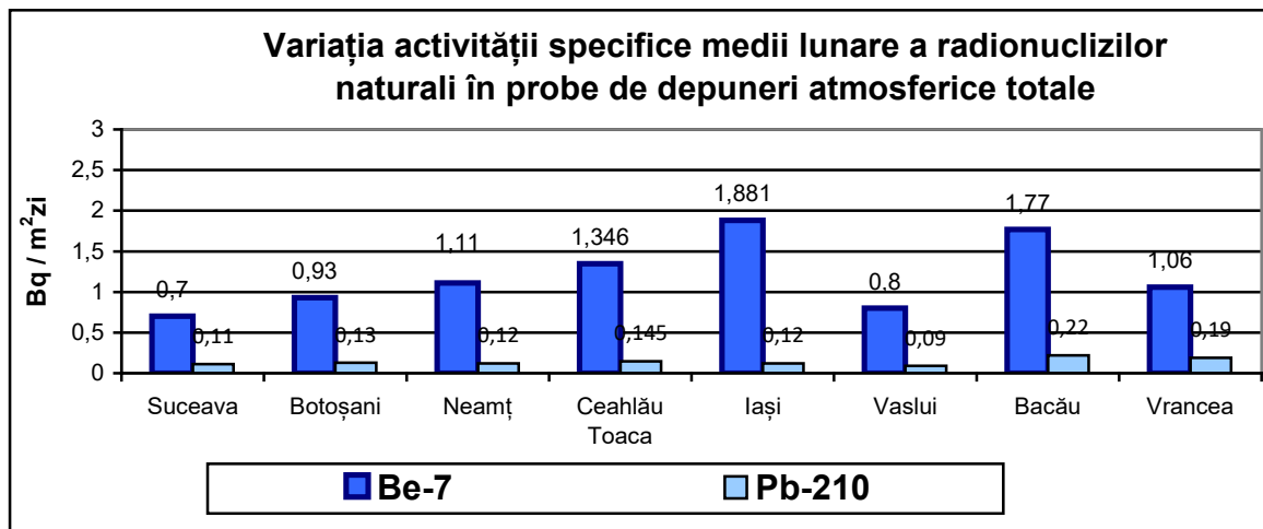
Figura IX.1.1.9. Variația activității specifice medii lunare a radionuclizilor naturali în probele de depuneri atmosferice totale, în anul de raportare 2020:
