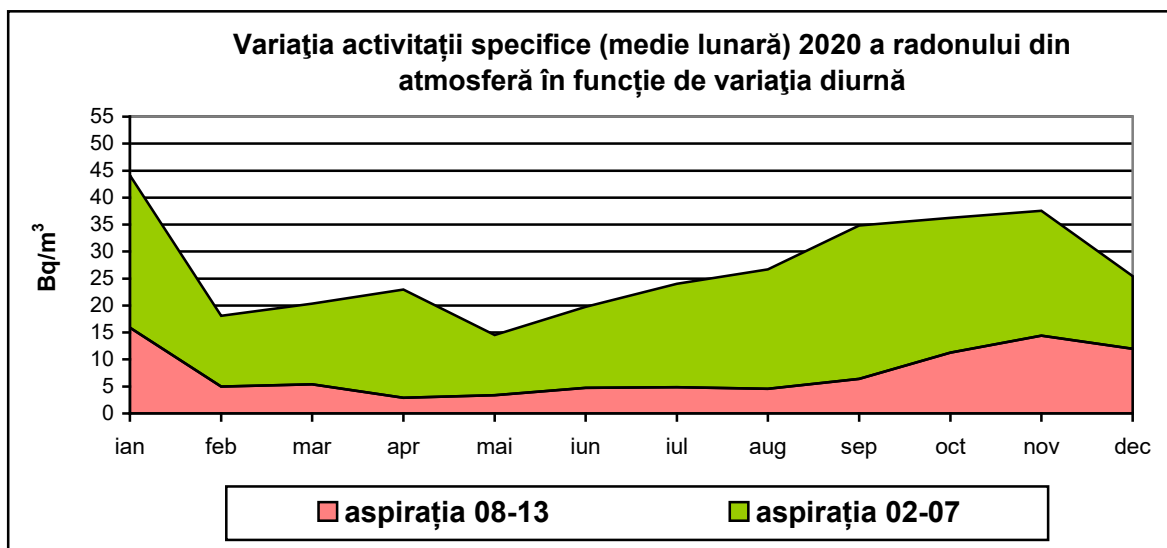
Figura IX.1.1.3. Variația activității specifice (medie lunară) 2020 a Radonului din atmosferă în funcție de variația diurnă
