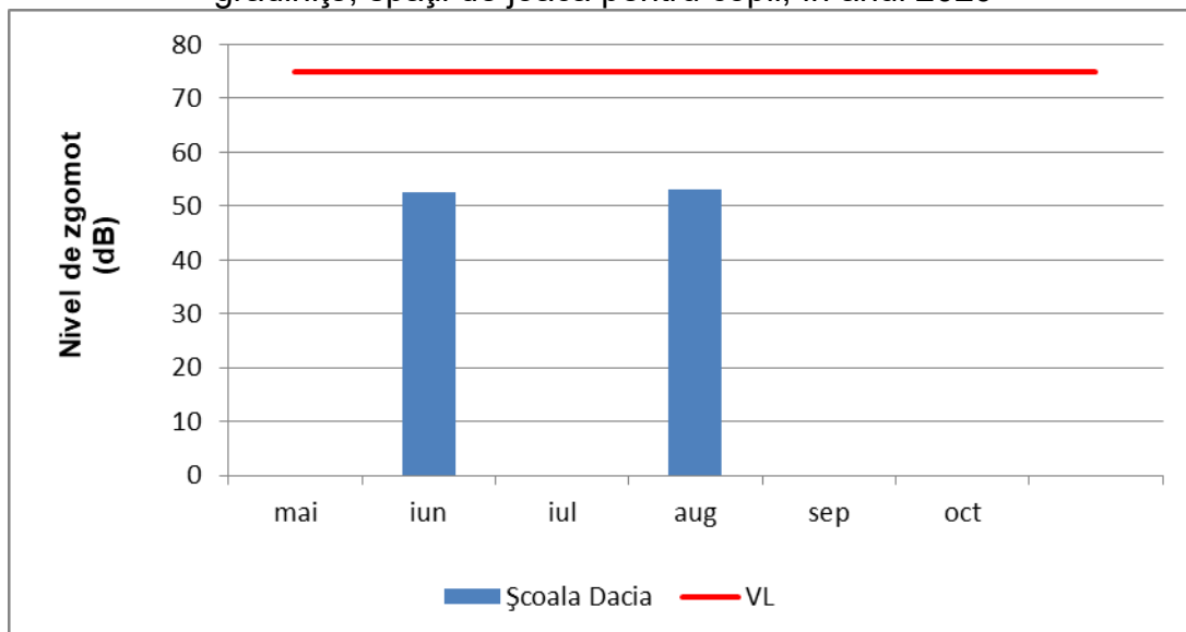
Figura VIII.1.2.1.10. Nivel de zgomot echivalent măsurat la limită - incinte de școli, creșe, grădinițe, spații de joacă pentru copii, în anul 2020
