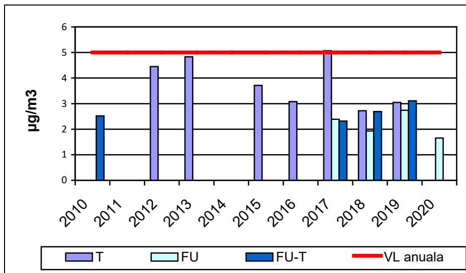
Figura I.1.1.2.5. C 6 H 6 – Evoluția concentrațiilor medii anuale înregistrate la stațiile de monitorizare în raport cu VL anuală, în perioada 2010 – 2020
