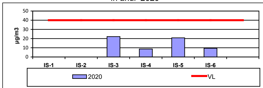
Figura I.1.1.1.1. NO 2 - Concentrațiile medii anuale înregistrate la stațiile de monitorizare, în anul 2020
