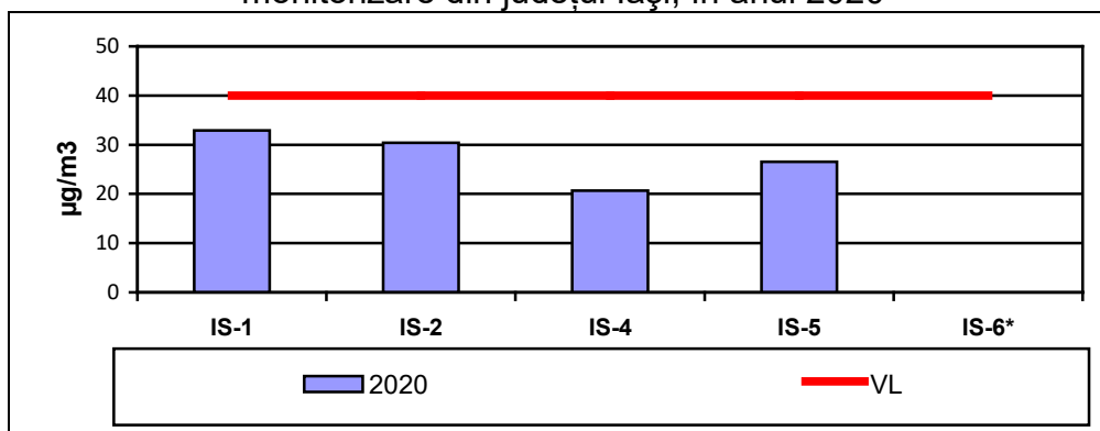
Figura I.1.1.1.3. PM10 gravimetric - Concentrațiile medii anuale înregistrate la stațiile de monitorizare din județul Iași, în anul 2020
