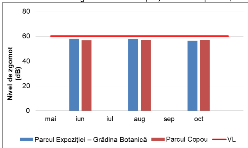
Figura VIII.1.2.1.1. Nivel de zgomot echivalent (dB) măsurat în parcuri, în anul 2020
