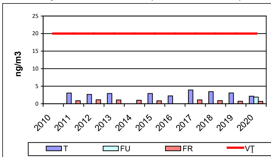
Figura I.1.1.2.8. Ni gravimetric determinat din fracția PM10 – Evoluția concentrațiilor medii anuale înregistrate la stațiile de monitorizare în raport cu VL anuală, în perioada 2010 – 2020
