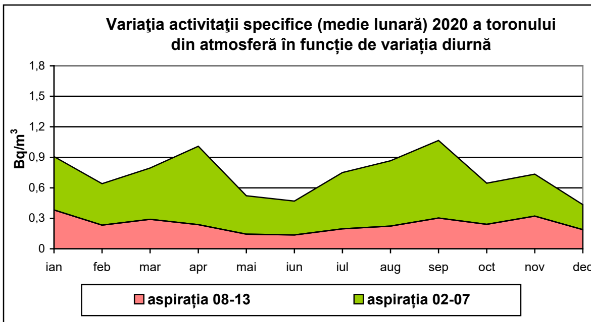
Figura IX.1.1.4. Variația activității specifice (medie lunară) 2020 a toronului din atmosferă în funcție de variația diurnă
