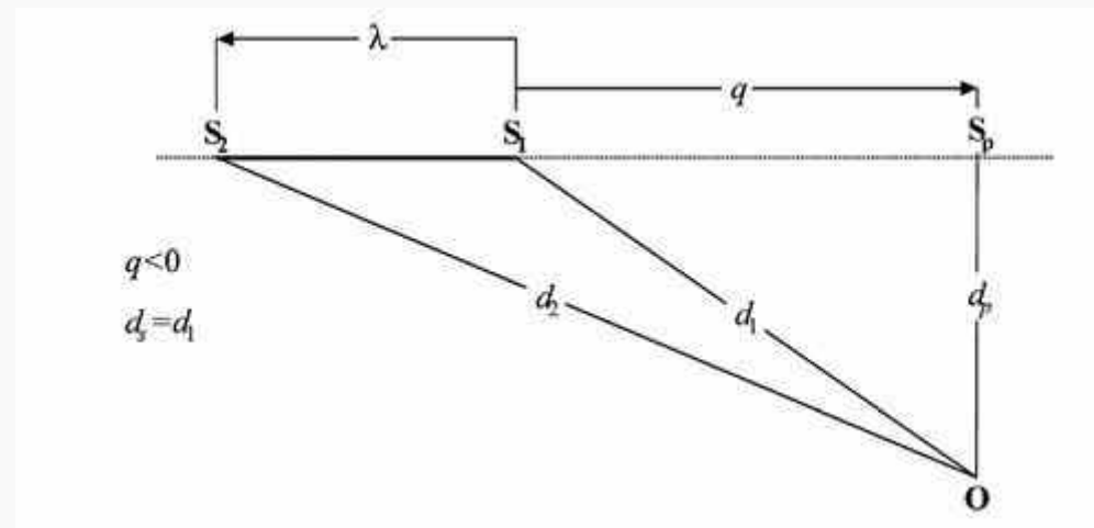
Figura 2.7.k: Geometria segmentului traiectului de zbor pentru poziția observatorului în dreptul segmentului
