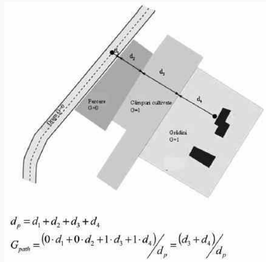
Figura 2.5.b: Determinarea coeficientului solului G_{path} pe o cale de propagare
