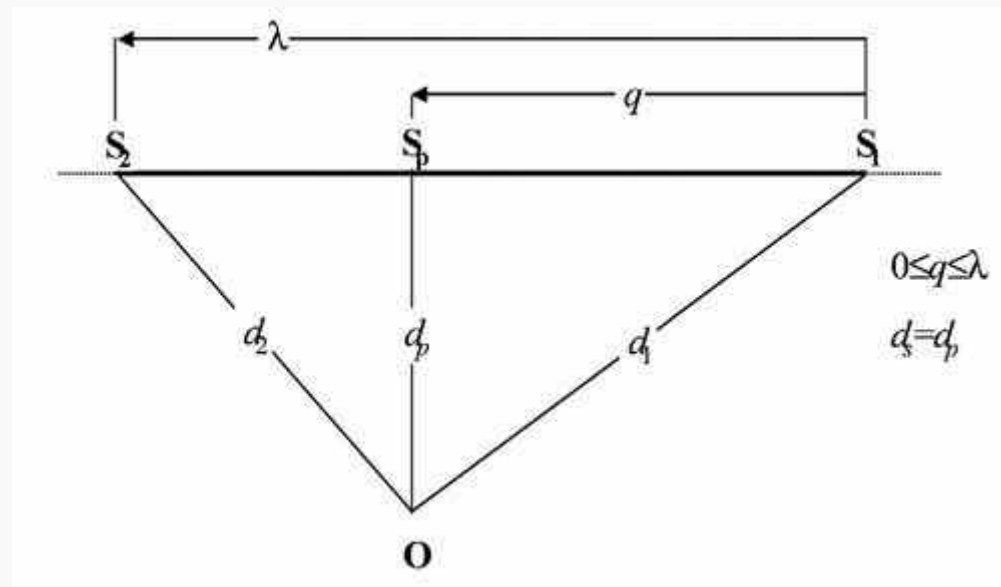
Figura 2.7.I: Geometria segmentului traiectului de zbor pentru poziția observatorului înaintea segmentului
