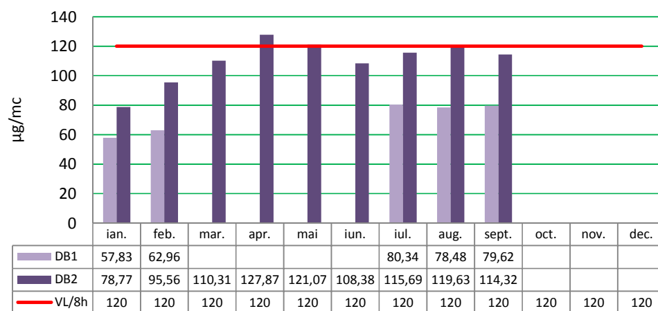
Valorile maxime/8h înregistrate pentru poluantul O 3 , comparate cu valoarea limită
