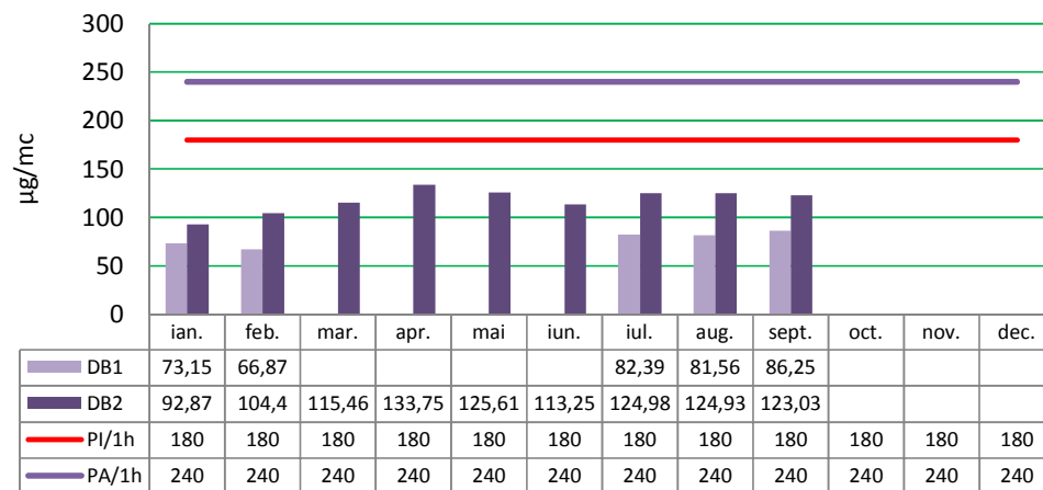
Valorile maxime/1h înregistrate pentru poluantul O 3 , comparate cu pragul de informare și pragul de alertă
