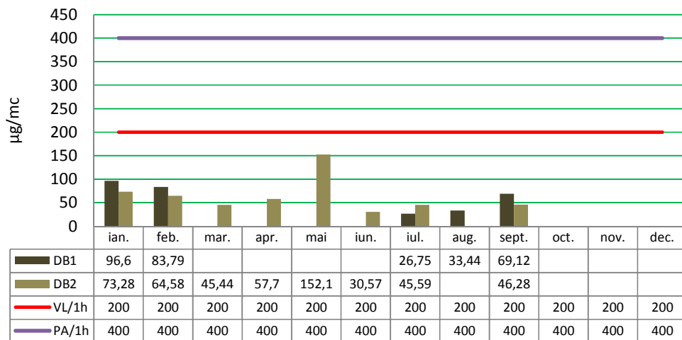
Valorile maxime/1h înregistrate pentru poluantul NO 2 , comparate cu valoarea limită și pragul de alertă
