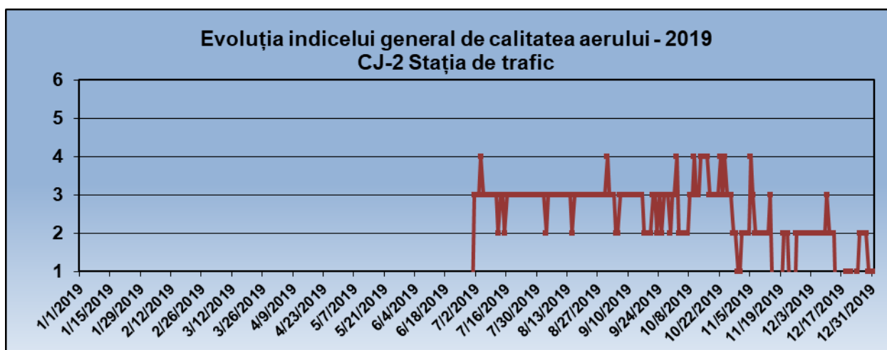
Figura 4.4. Evoluția indicelui general de calitatea aerului, stația de tip suburban (CJ-2) din Cluj-Napoca în anul 2019
