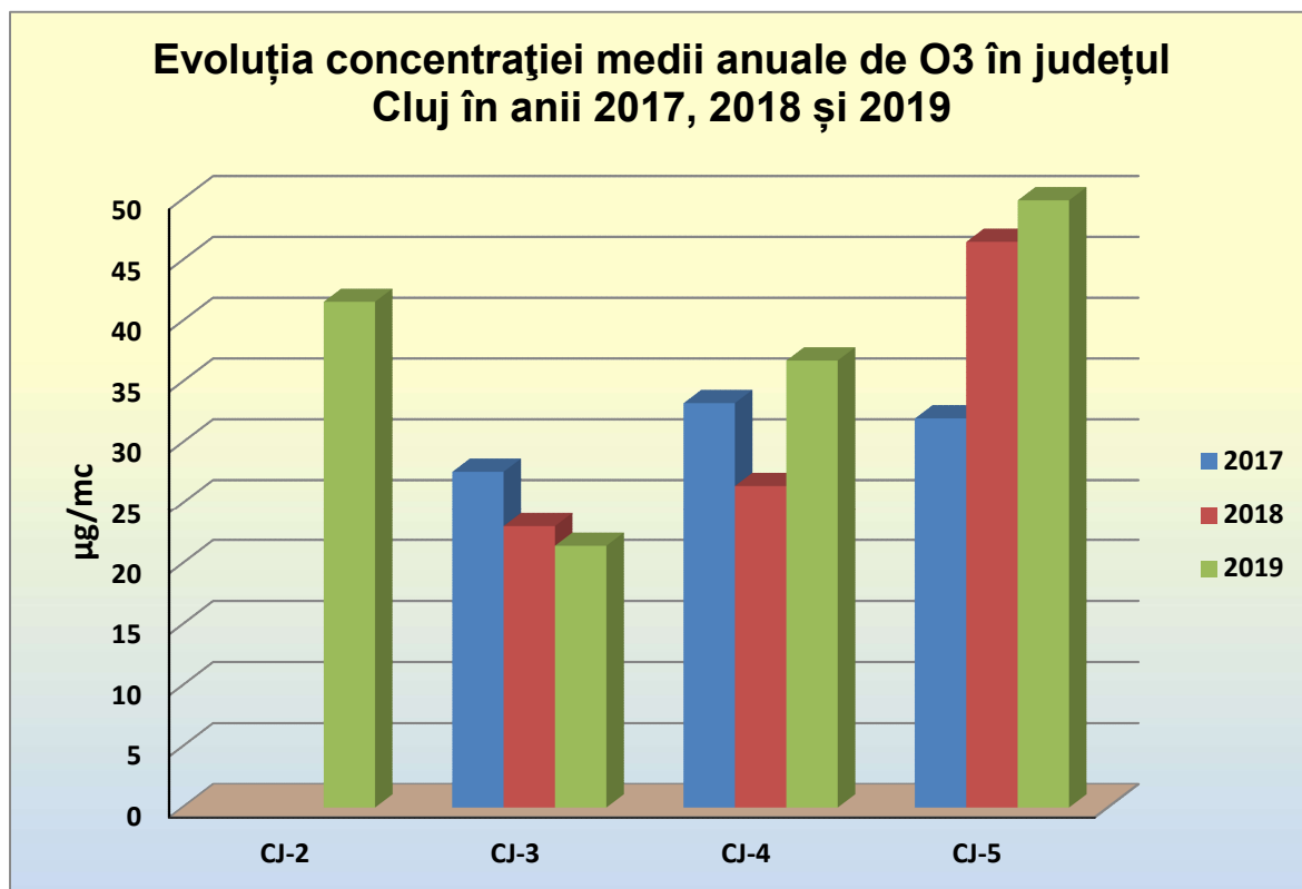
Figura 2.4.3. Evoluția concentrațiilor medii anuale pentru indicatorul O 3 , județul Cluj în anii 2017, 2018 și 2019
