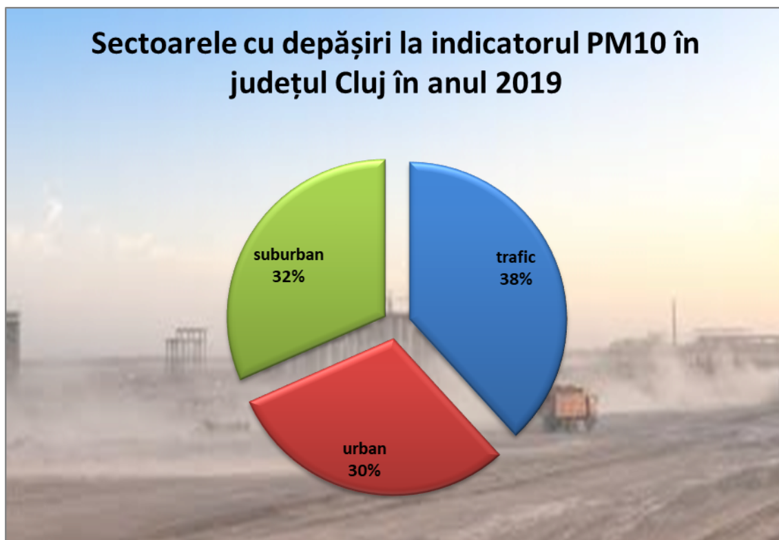
Figura 2.5.2.2. Sectoarele cu depășiri la indicatorul PM 10 , în județul Cluj, în anul 2019.
