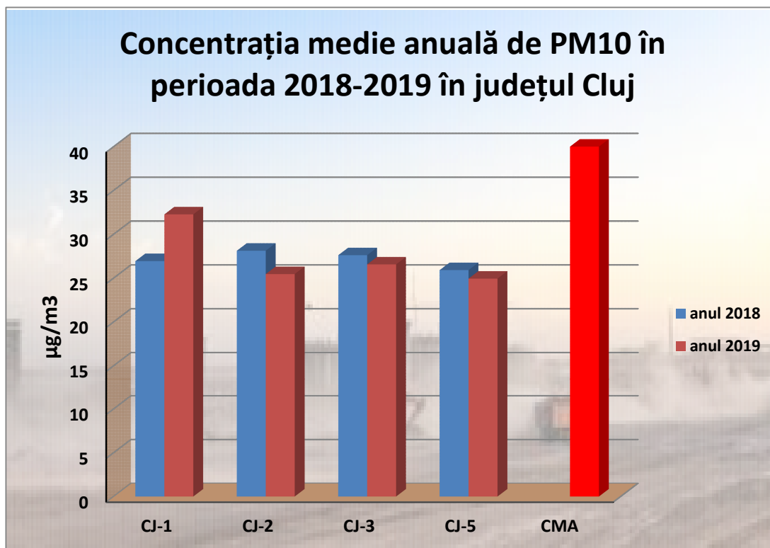
Figura 2.5.2.5. Evoluția concentrațiilor medii anuale pentru indicatorul PM 10 , județul Cluj în perioada 2018-2019.
