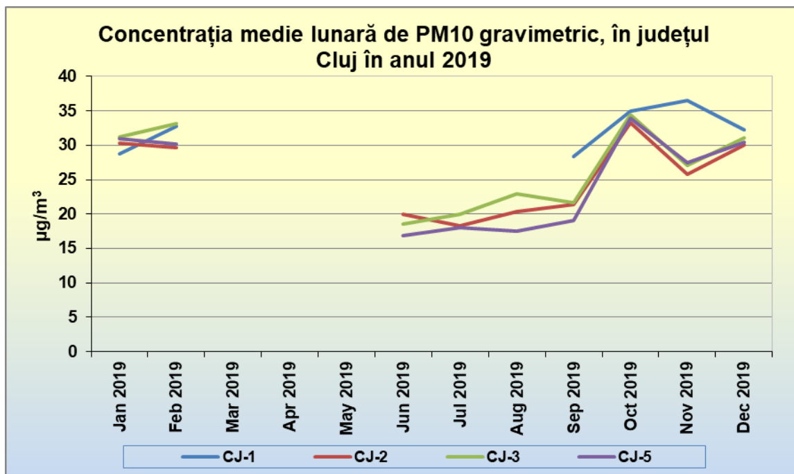
Figura 2.5.2.1. Evoluția concentrațiilor medii lunare pentru indicatorul PM 10 , în județul Cluj, în anul 2019 (metoda gravimetrică).
