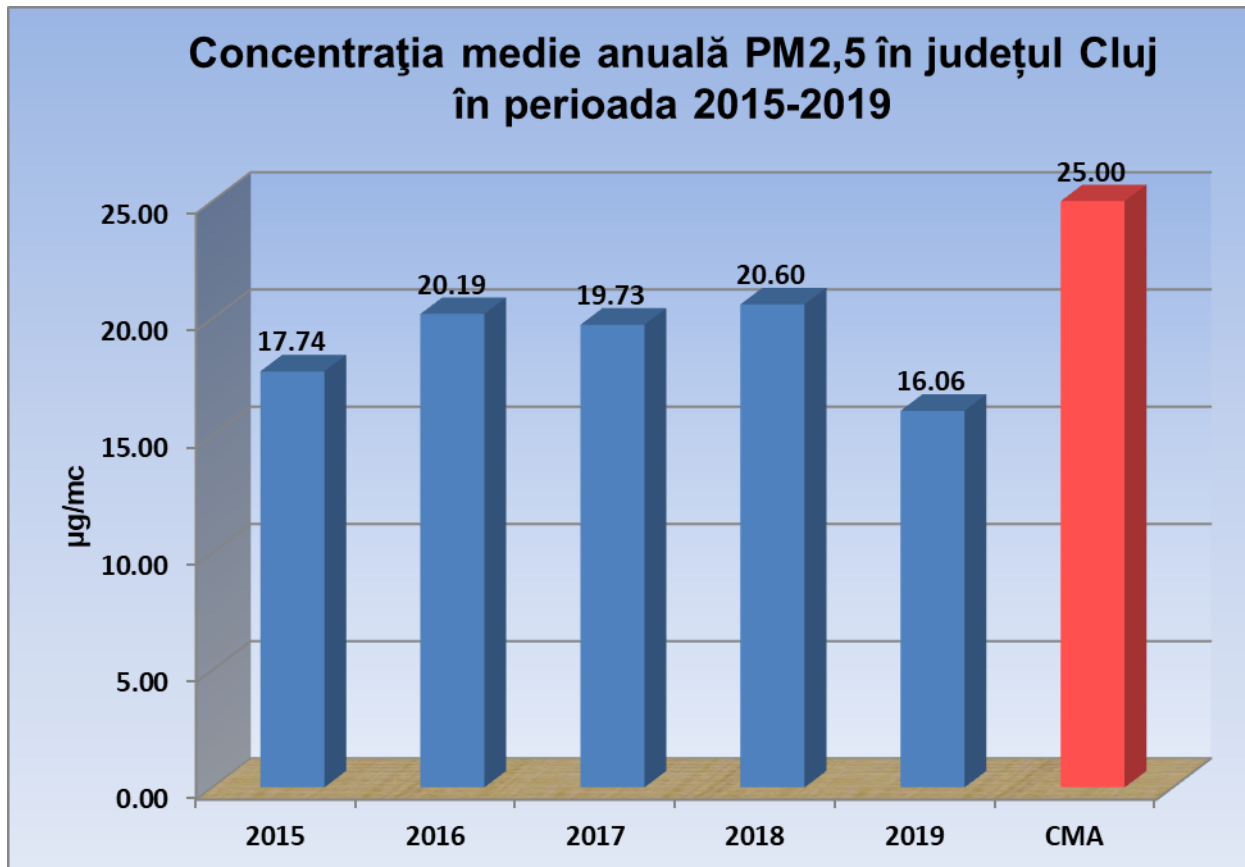
Figura 2.5.1.2. Evoluția concentrațiilor medii anuale pentru indicatorul PM_{2,5} , județul Cluj, în perioada 2015-2019
