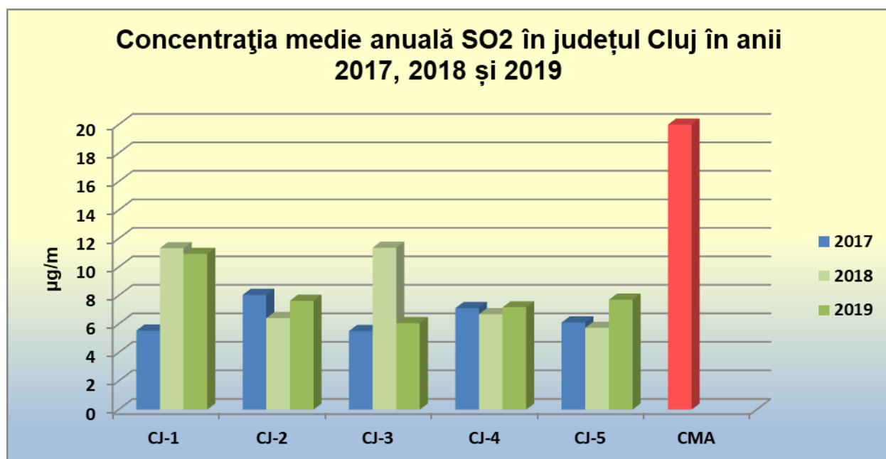
Figura 2.1.1.3. Evoluția concentrațiilor medii anuale pentru indicatorul SO 2 , județul Cluj în anii 2017, 2018 și 2019
