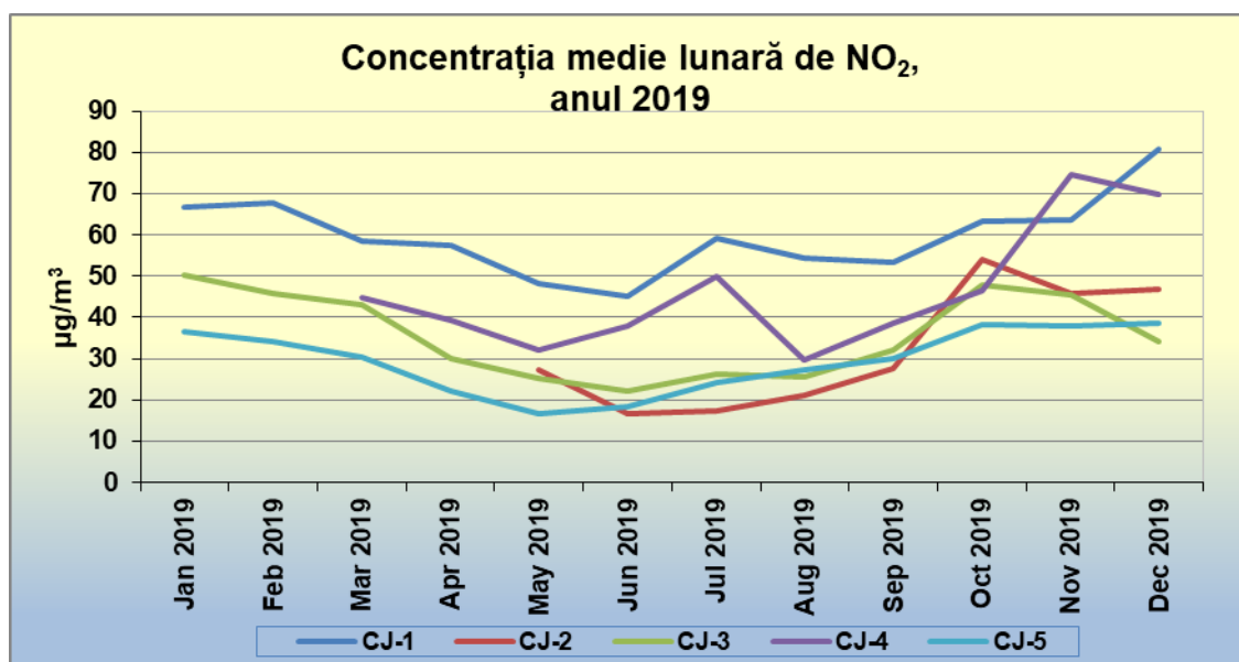
Figura 2.2.1.1. Evoluția concentrațiilor medii lunare pentru indicatorul \text{NO}_2 , județul Cluj, din anul 2019
