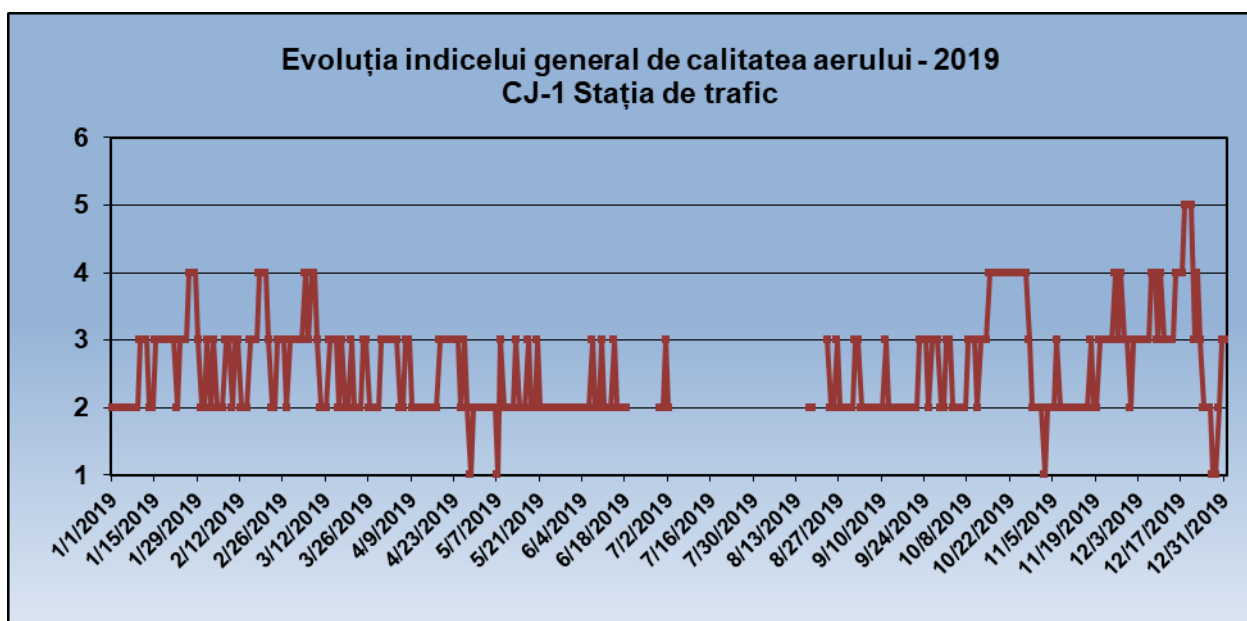
Figura 4.2. Evoluția indicelui general de calitate a aerului, stația de tip trafic (CJ-1) din Cluj-Napoca în anul 2019
