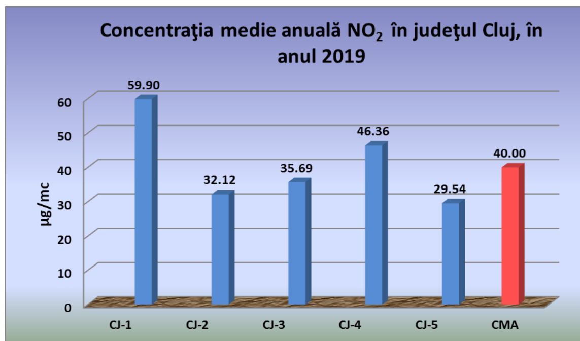
Figura 2.2.1.2. Evoluția concentrațiilor medii anuale pentru indicatorul NO 2 , județul Cluj, 2019
