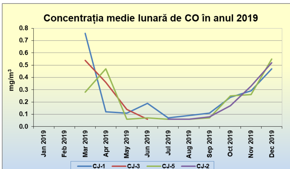
Figura 2.3.1. Evoluția concentrațiilor medii lunare pentru indicatorul CO, județul Cluj, 2019
