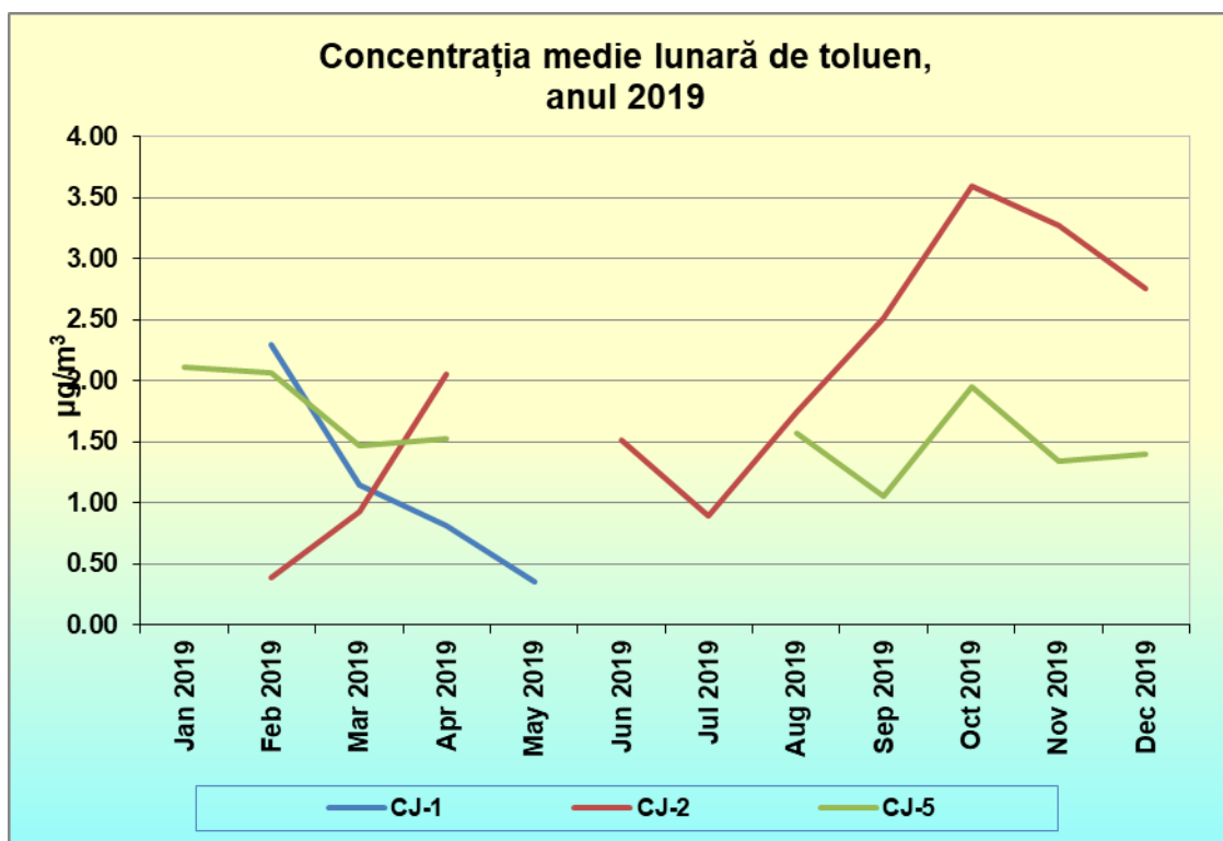
Figura 2.7.3. Variația concentrației medii lunare de toluen în anul 2019 în județul Cluj
