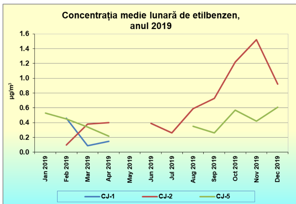
Figura 2.7.4. Variația concentrației medii lunare de etilbenzen în anul 2019 în județul Cluj
