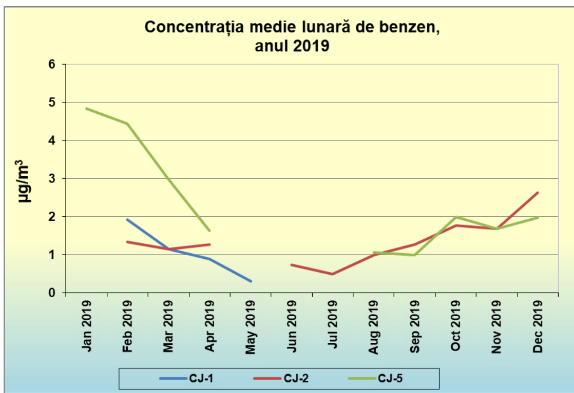
Figura 2.7.1. Variația concentrației medii lunare de benzen în anul 2019 în județul Cluj
