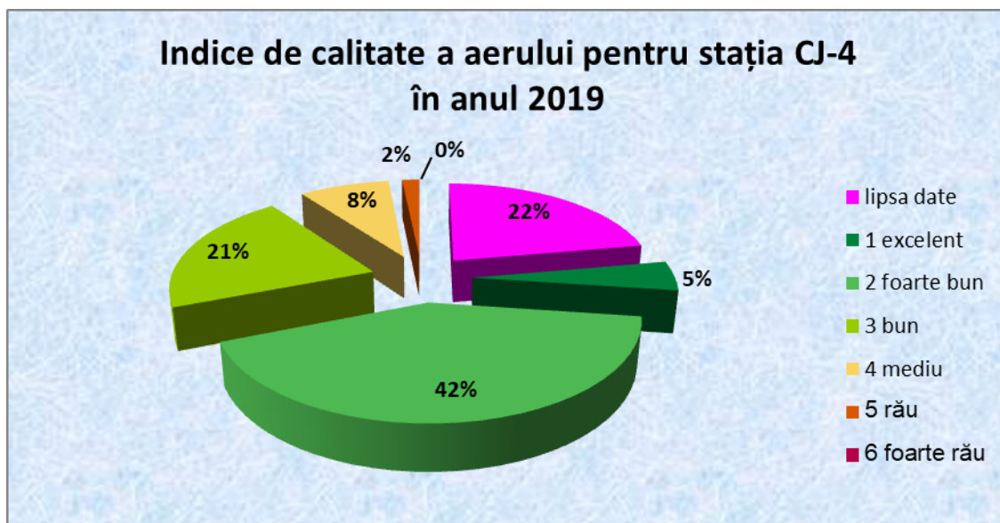
Figura 4.9. Indicele general de calitate a aerului, la stația CJ-4 în anul 2019
