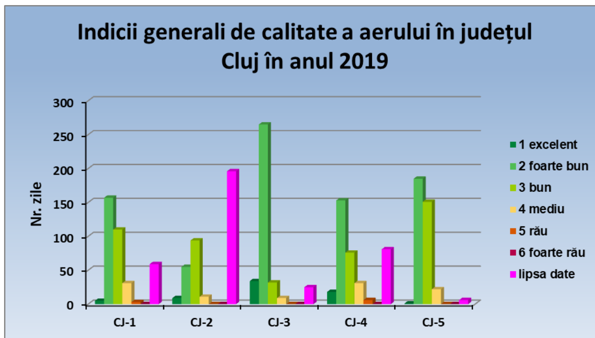
Figura 4.12. Indicii generali de calitate a aerului la stațiile de monitorizare automate a aerului din județul Cluj în anul 2019
