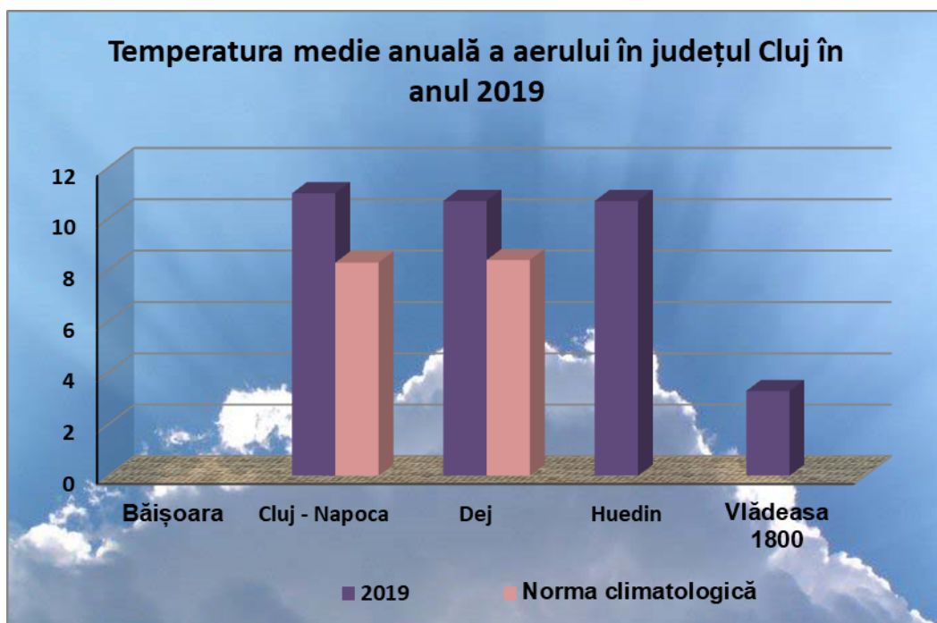
Figura 1.8. Evoluția temperaturilor medii anuale în județul Cluj în anul 2019
