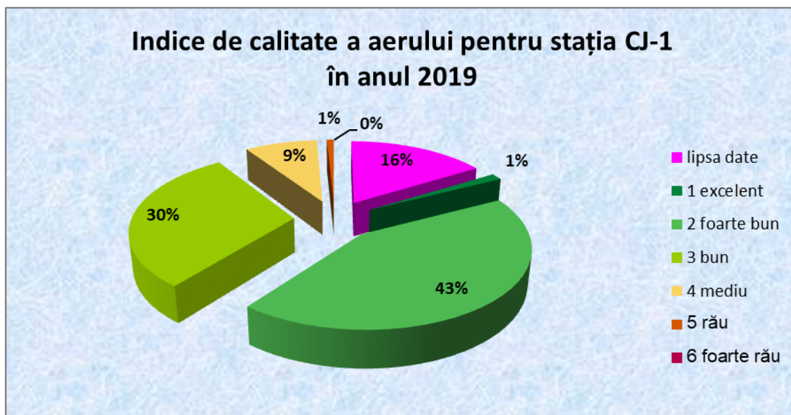
Figura 4.3. Indicele general de calitatea aerului, la stația CJ-1 în anul 2019
