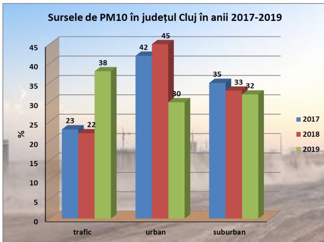
Figura 2.5.2.3. Sursele de PM 10 , în județul Cluj, în perioada 2017- 2019.
