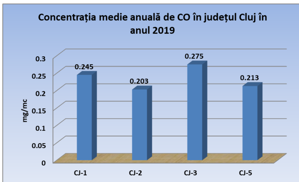
Figura 2.3.2. Valoarea concentrațiilor medii anuale pentru indicatorul CO, în județul Cluj, în anul 2019
