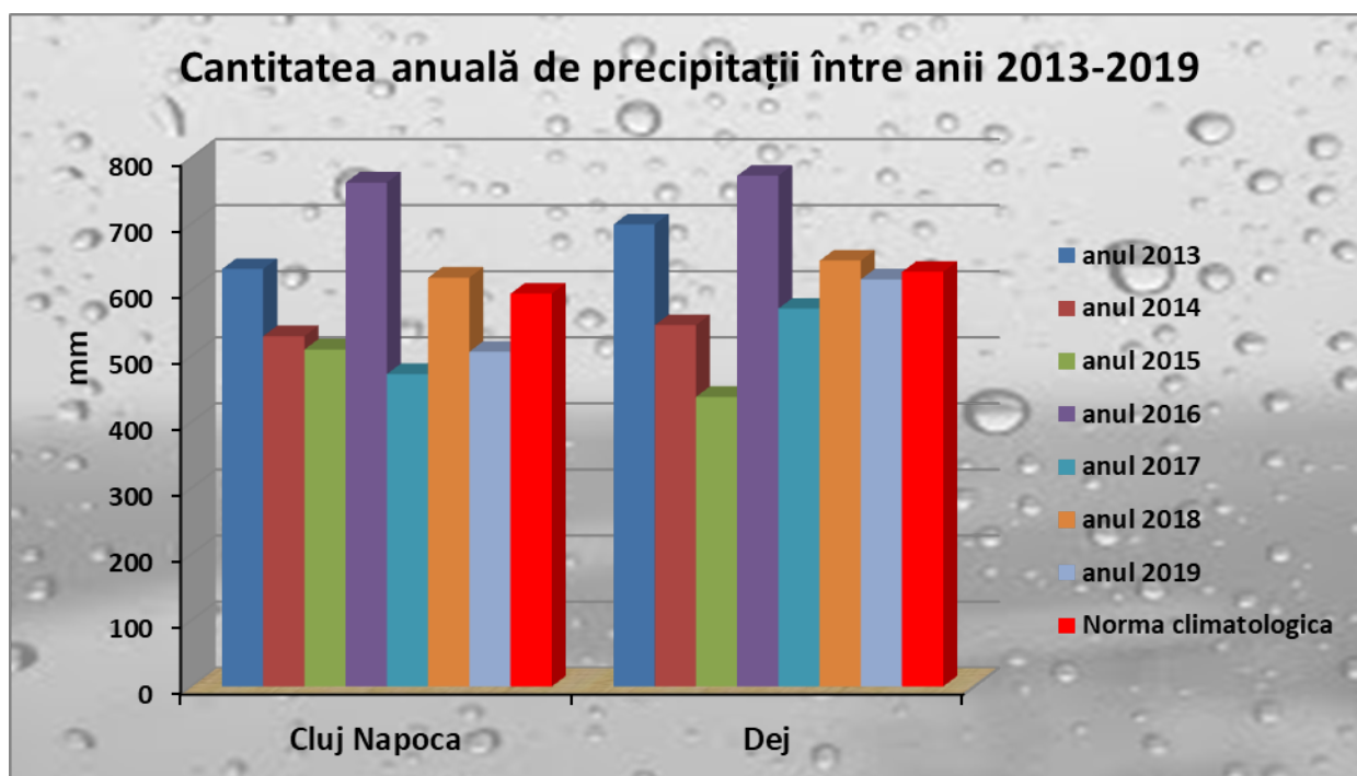
Figura 1.11. Evoluția precipitațiilor medii anuale în județul Cluj în perioada 2013 - 2019
