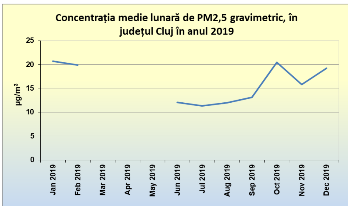
Figura 2.5.1.1. Evoluția concentrațiilor medii lunare pentru indicatorul PM_{2,5} , județul Cluj, în anul 2019
