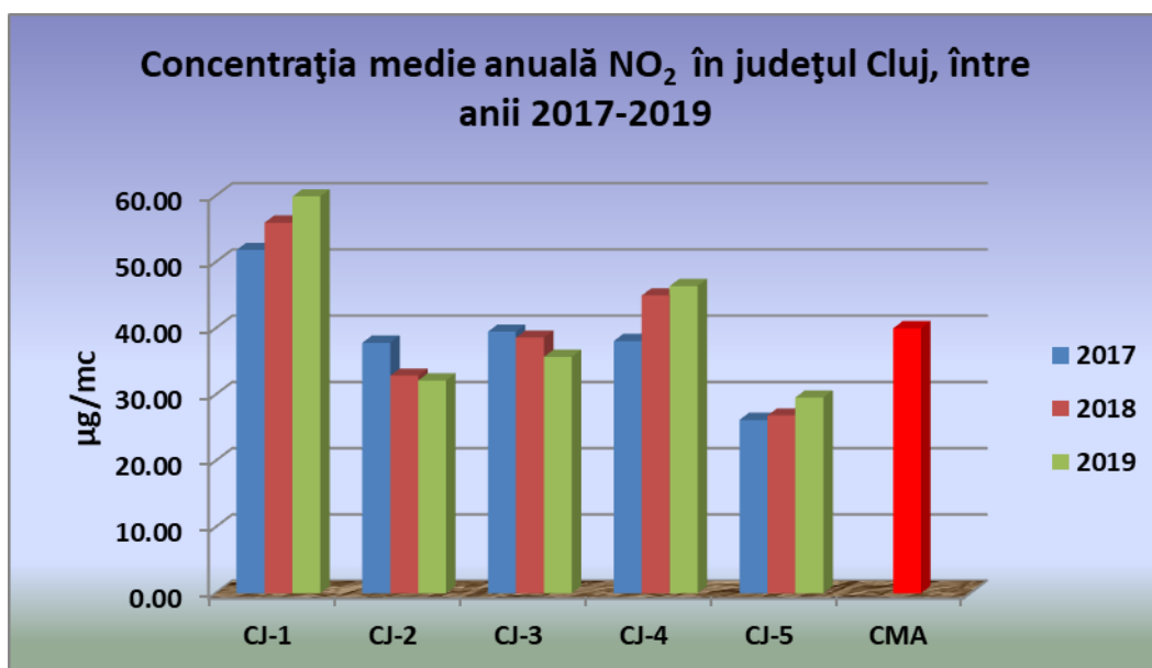
Figura 2.2.1.3. Evoluția concentrațiilor medii anuale pentru indicatorul NO 2 , județul Cluj, în anii 2017 – 2019
