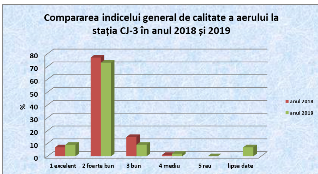
Figura 4.14. Compararea indicelui general de calitatea aerului la stația CJ-3 în anii 2018 și 2019
