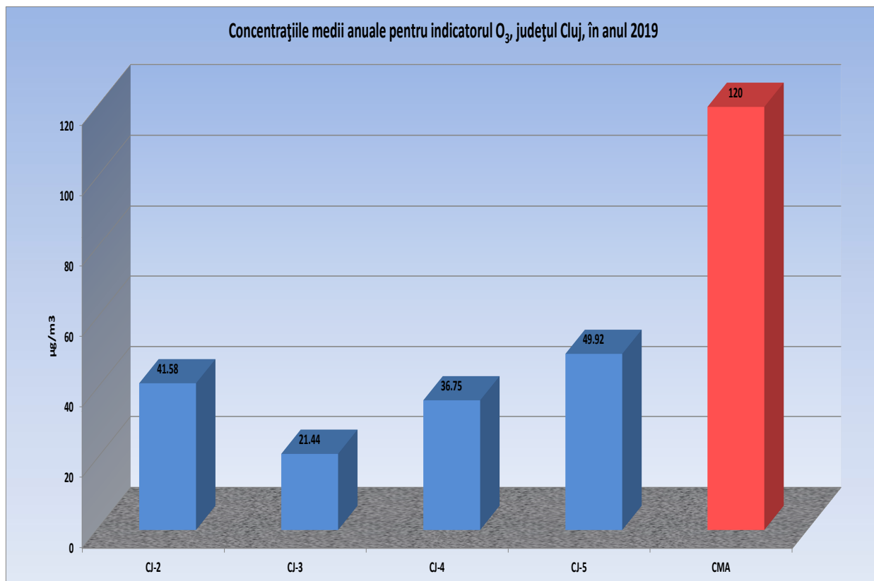
Figura 2.4.2. Evoluția concentrațiilor medii anuale pentru indicatorul O 3 , județul Cluj, în anul 2019
