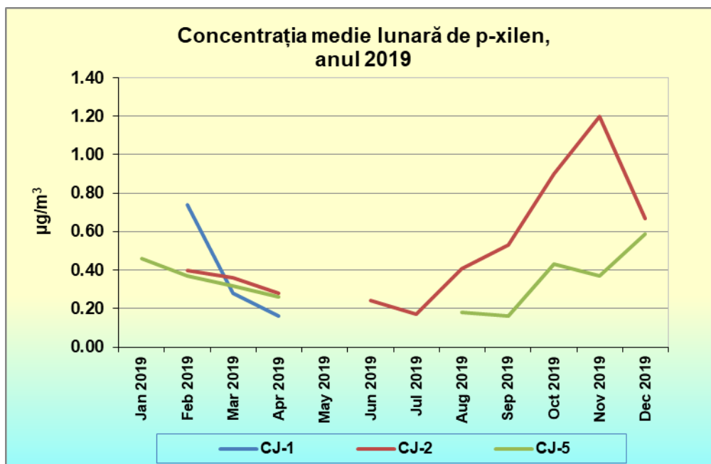
Figura 2.7.7. Variația concentrației medii lunare de p-xilen în anul 2019 în județul Cluj
