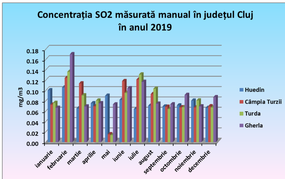
Figura 2.1.2.1 Evoluția concentrației medii de dioxid de sulf din aer măsurată manual cu metoda de scurtă durată (MSD) în județul Cluj în anul 2019.
