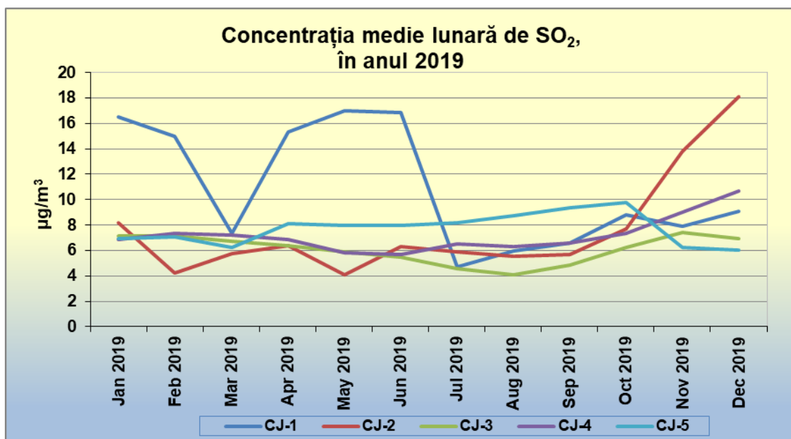
Figura 2.1.1.1. Evoluția concentrațiilor medii lunare pentru indicatorul SO 2 , județul Cluj, din anul 2019
