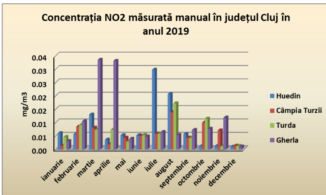
Figura 2.2.2.1 Evoluția concentrației medii de dioxid de azot din aer măsurată manual cu metoda de scurtă durată (MSD) în județul Cluj în anul 2019.
