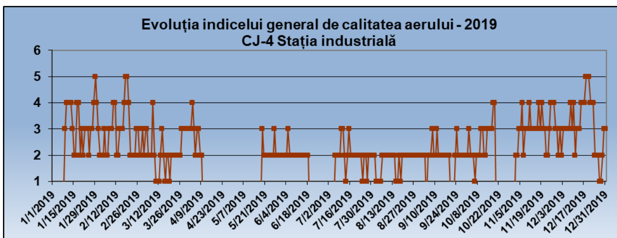
Figura 4.8. Evoluția indicelui general de calitatea aerului, stația de tip industrial (CJ-4) din Cluj-Napoca în anul 2019
