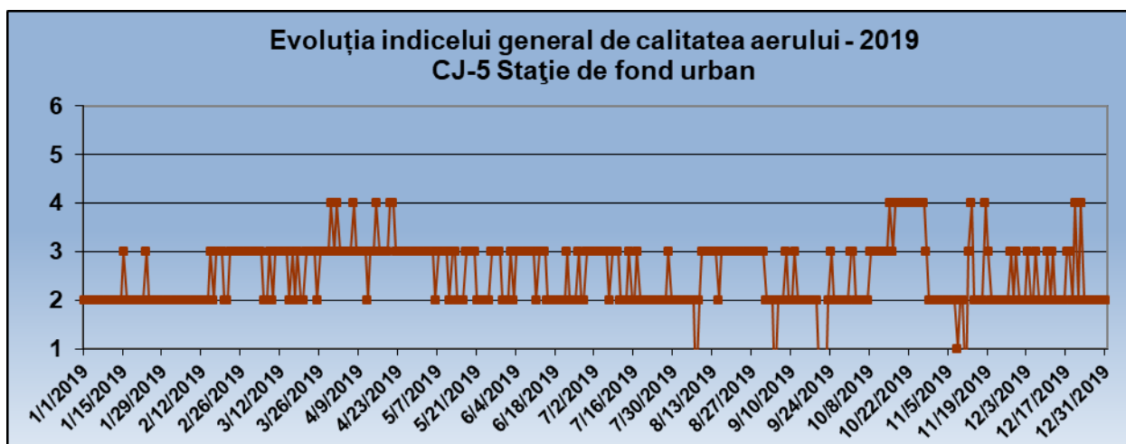
Figura 4.10. Evoluția indicelui general de calitate a aerului, municipiul Dej, 2019
