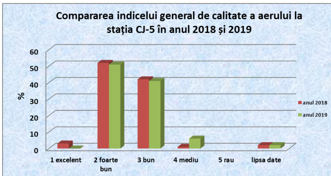
Figura 4.16. Compararea indicelui general de calitatea aerului la stația CJ-5 în anii 2018 și 2019
