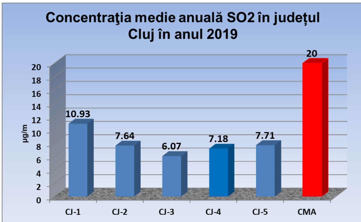
Figura 2.1.1.2. Evoluția concentrațiilor medii anuale pentru indicatorul SO 2 , județul Cluj, 2019
