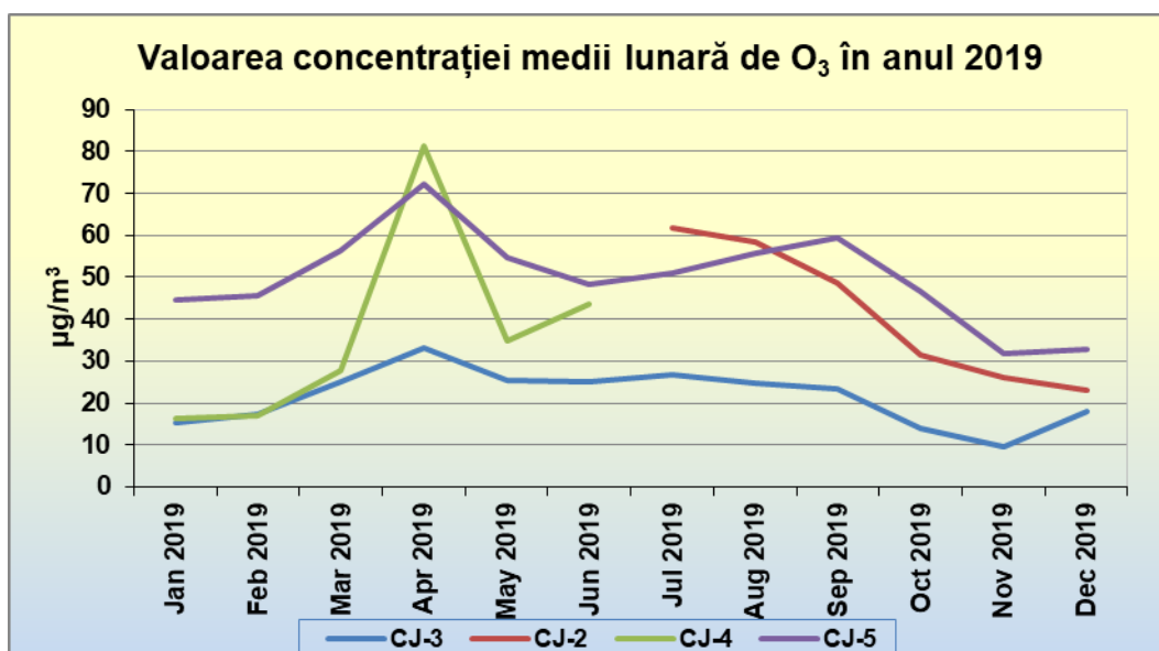
Figura 2.4.1. Evoluția concentrațiilor medii lunare pentru indicatorul O 3 , județul Cluj, din anul 2019
