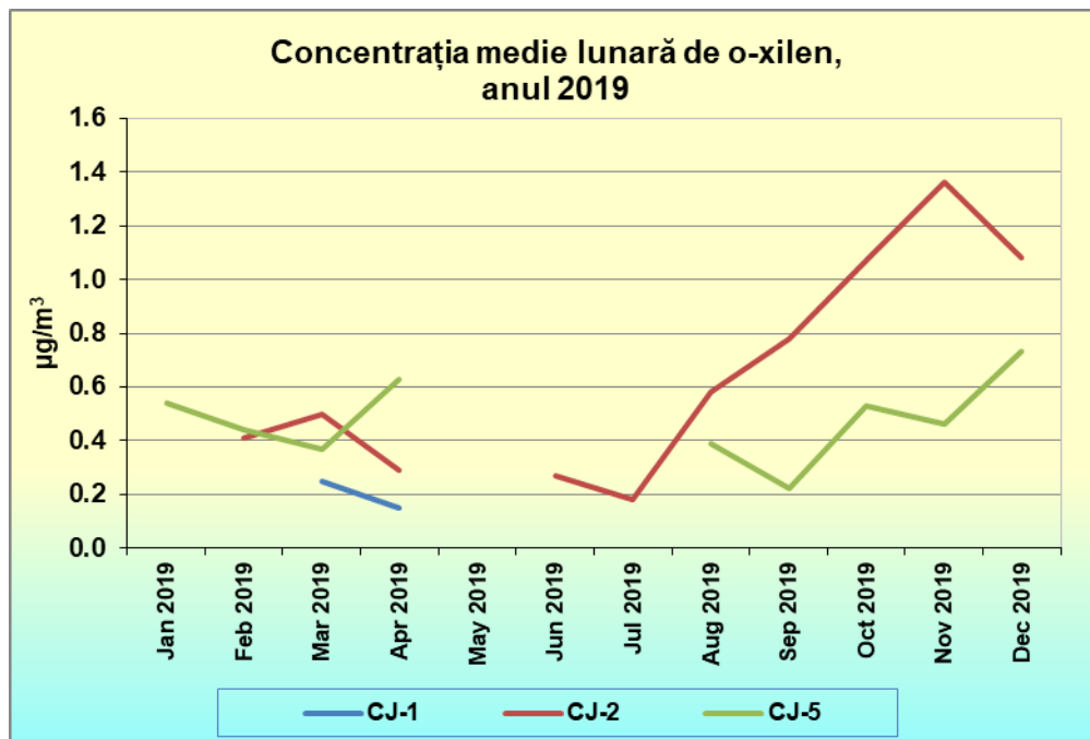
Figura 2.7.5. Variația concentrației medii lunare de o-xilen în anul 2019 în județul Cluj
