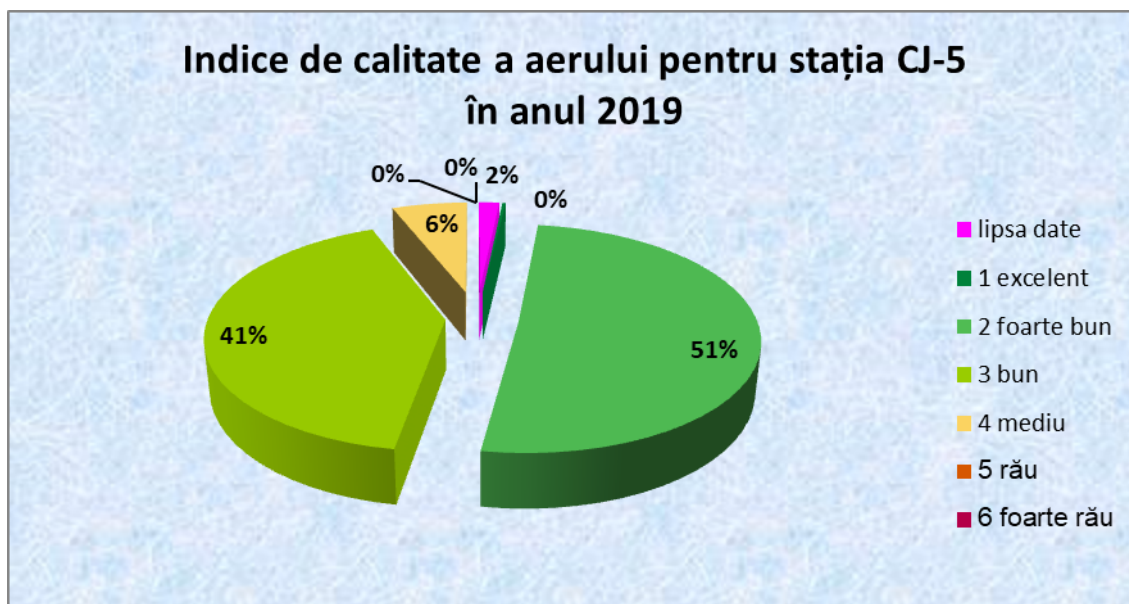
Figura 4.11. Indicelui general de calitate a aerului, municipiul Dej, 2019
