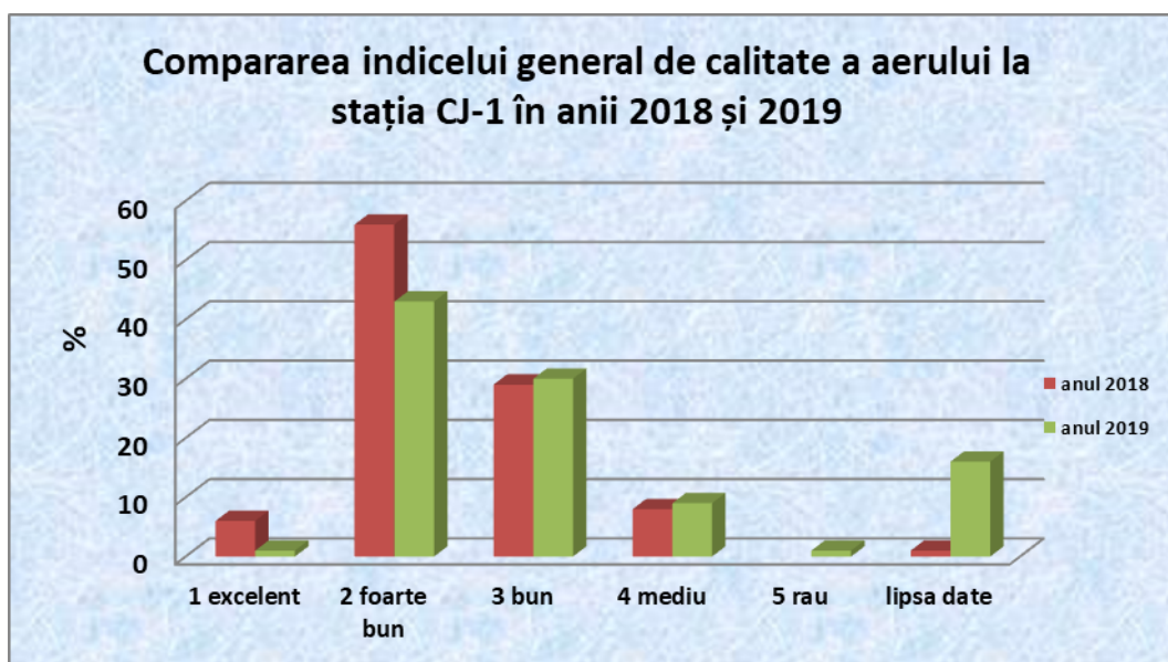
Figura 4.13. Compararea indicelui general de calitatea aerului la stația CJ-1 în anii 2018 și 2019
