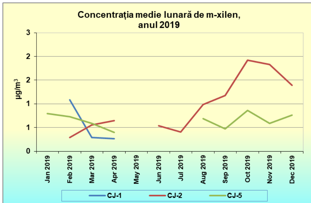
Figura 2.7.6. Variația concentrației medii lunare de m-xilen în anul 2019 în județul Cluj
