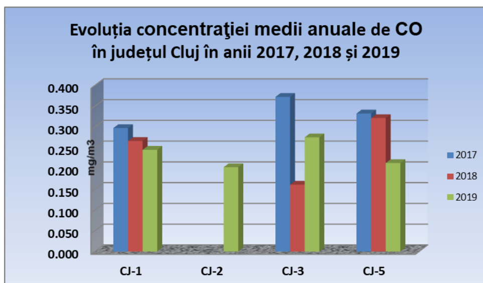
Figura 2.3.3. Evoluția concentrațiilor medii anuale pentru indicatorul CO, județul Cluj, în anul 2019 comparativ cu 2017 și 2018.
