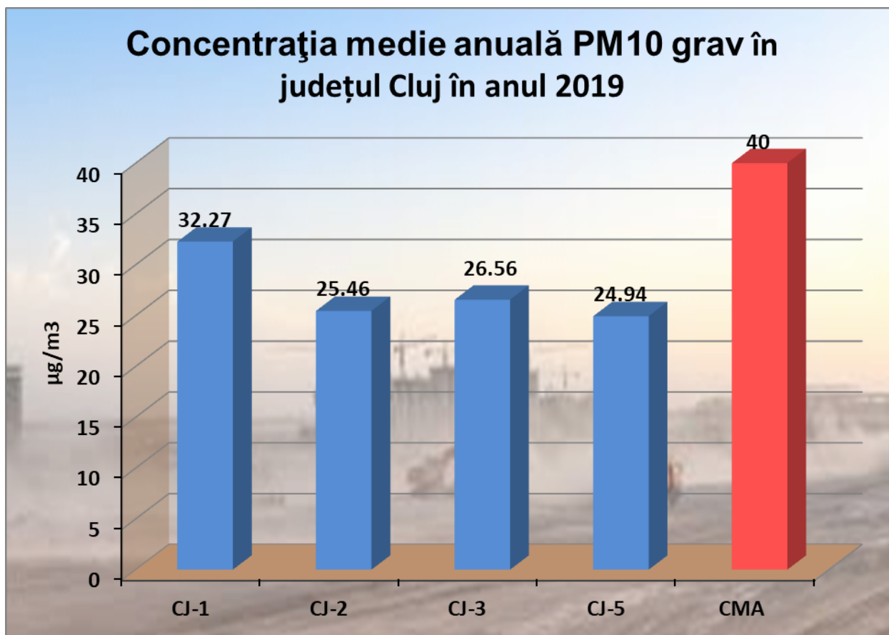
Figura 2.5.2.4. Evoluția concentrațiilor medii anuale pentru indicatorul PM 10 , județul Cluj, în anul 2019 (metoda gravimetrică)
