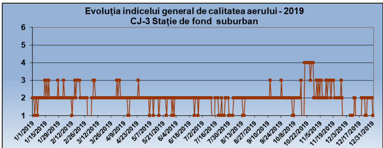
Figura 4.6. Evoluția indicelui general de calitatea aerului, stația de tip suburban (CJ-3) din Cluj-Napoca în anul 2019
