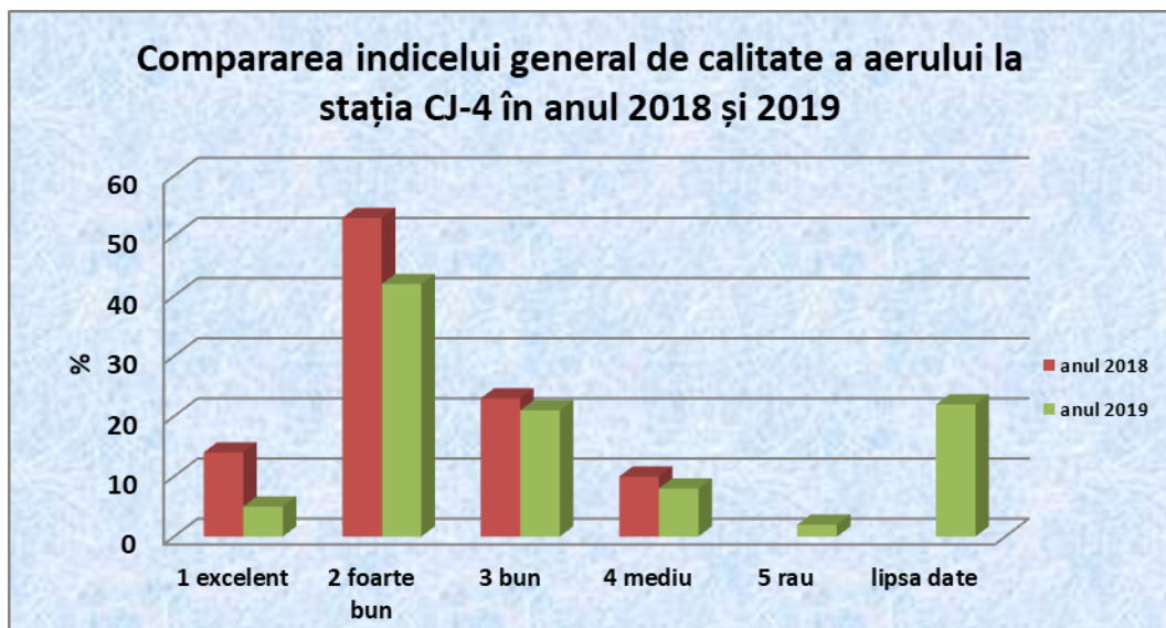
Figura 4.15. Compararea indicelui general de calitatea aerului la stația CJ-4 în anii 2018 și 2019
