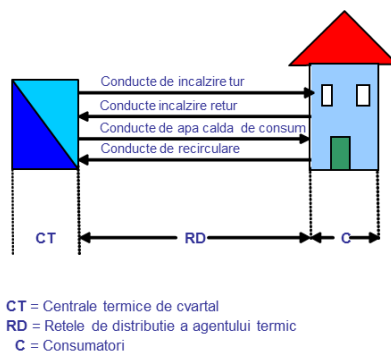
Fig. 2 Structura SACET - CTC
