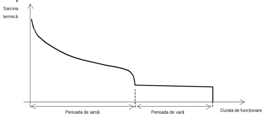
Fig. 6. Necesari de căldură – curba clasată
