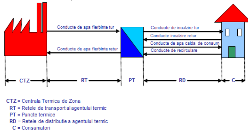
Fig. 4 Structura SACET – CTZ Someș Nord
