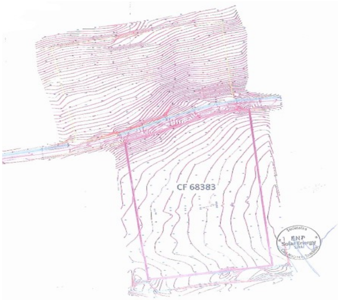
Fig.3.2 Plan topografic
