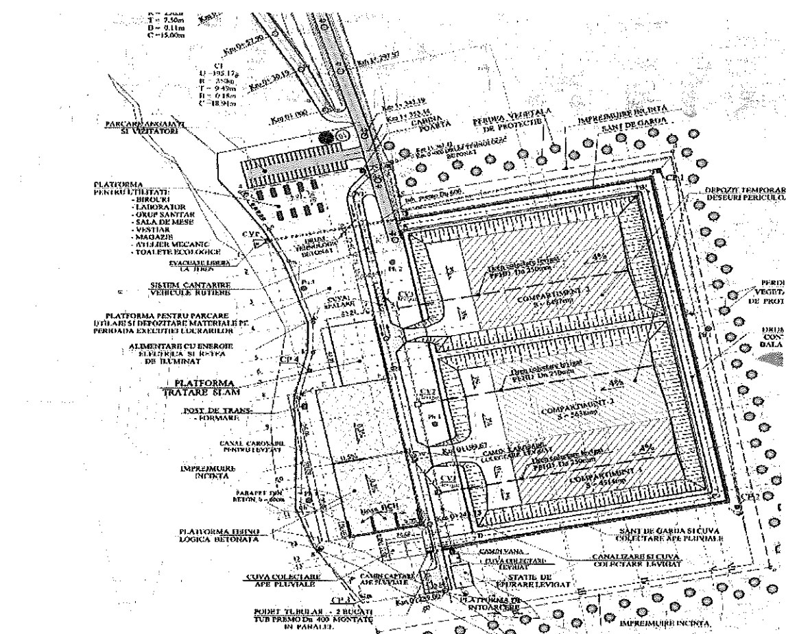
Figura 1 – organizare amplasament
